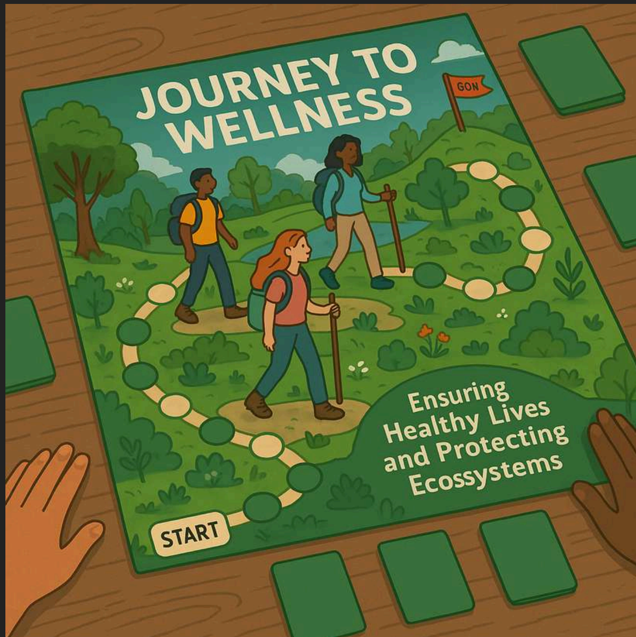
Chat GPT
