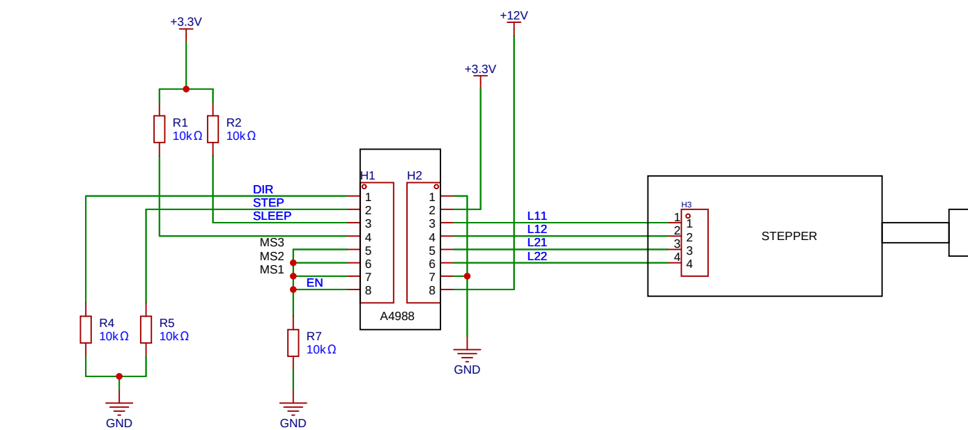
MOTOR DE PASSO (a4988)
