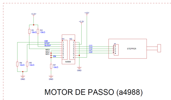
Como sistema motor do tapete da esteira, foi utilizado um motor de passo NEMA 22 controlado pelo driver A4988, conforme o esquemático da Fig. 8. Os pinos STEP, DIR e SLEEP são utilizados, respectivamente, para avançar um passo, definir a direção de rotação e habilitar ou desabilitar o driver (liberando ou travando o eixo). Esses componentes foram escolhidos por sua disponibilidade e pela baixa complexidade operacional do driver .
