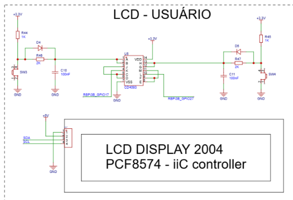
Figura 12. Esquemático do display LCD 2004 (PCF8574, I 2 C) e dos botões START/STOP com condicionamento CD4093.
