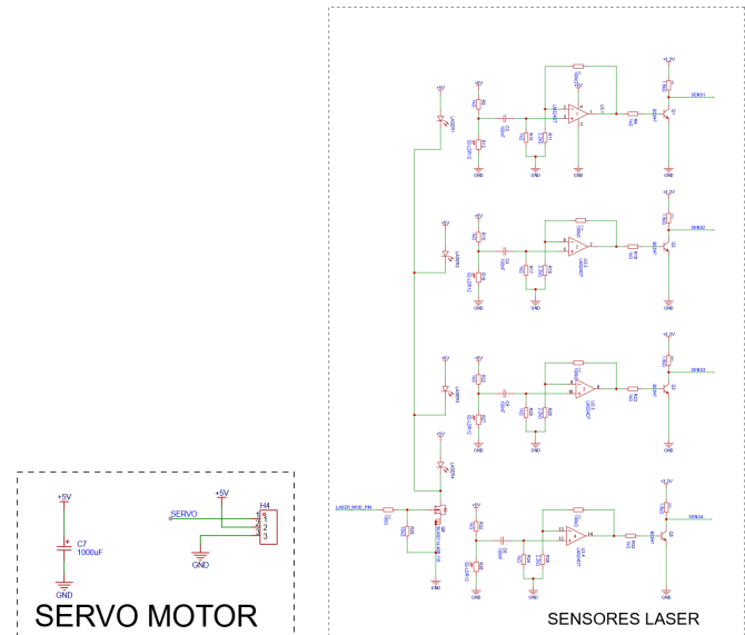
Figura 10. Esquemático dos quatro sensores laser com condicionamento de sinal (LDR + LM324).
