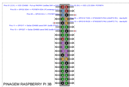
Figura 13. Esquemático de pinagem do header GPIO do Raspberry Pi 3B com as conexões do projeto (EasyEDA).
