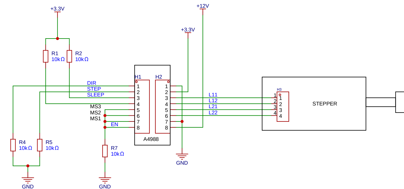
MOTOR DE PASSO (a4988)
