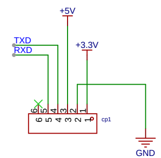
COMUNICAÇÃO UART <> USB
