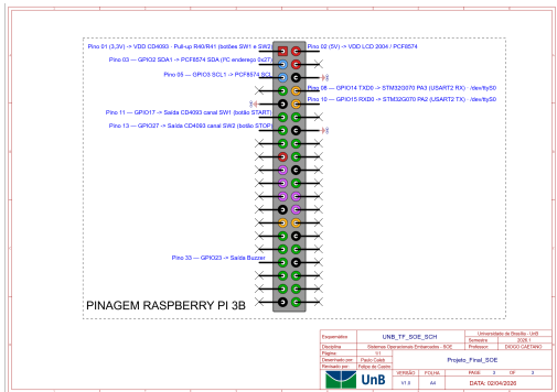
Figura 13. Esquemático de pinagem do header GPIO do Raspberry Pi 3B com as conexões do projeto (EasyEDA).
