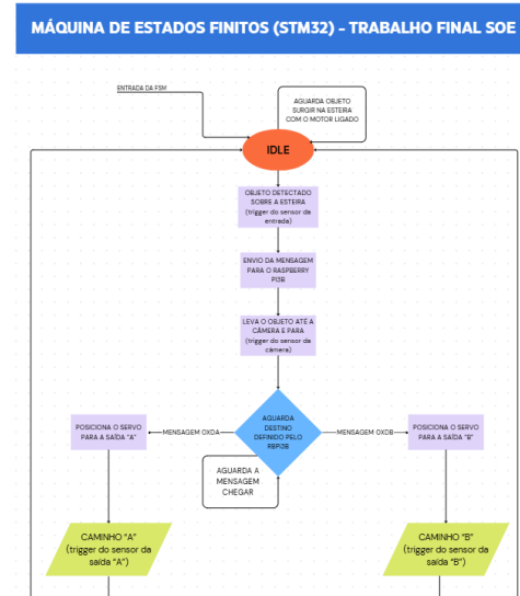
Figura 14. Diagrama de estados da FSM do firmware do STM32G070.
