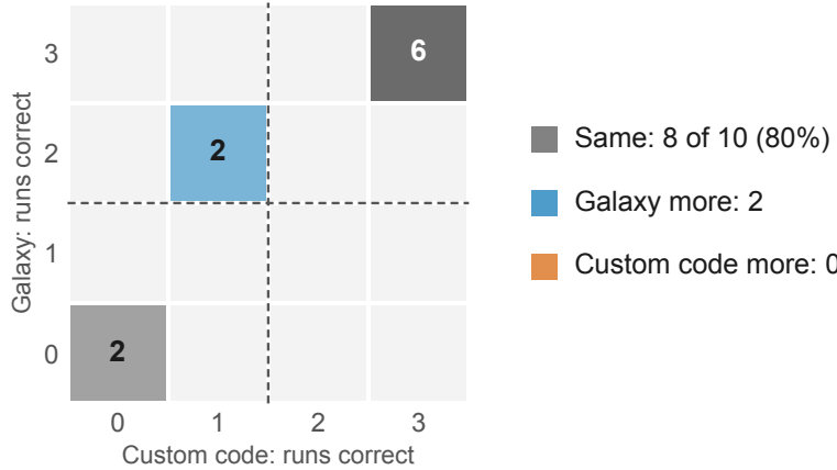
GPT-5.5
