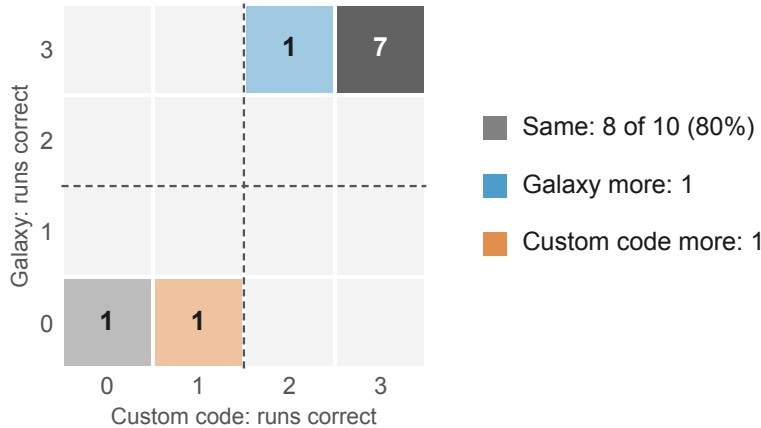
GPT-5.6 Sol
