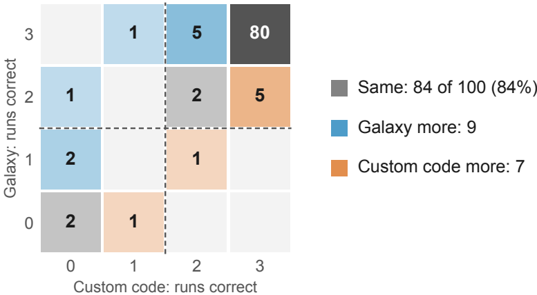
GPT-5.6 Sol
