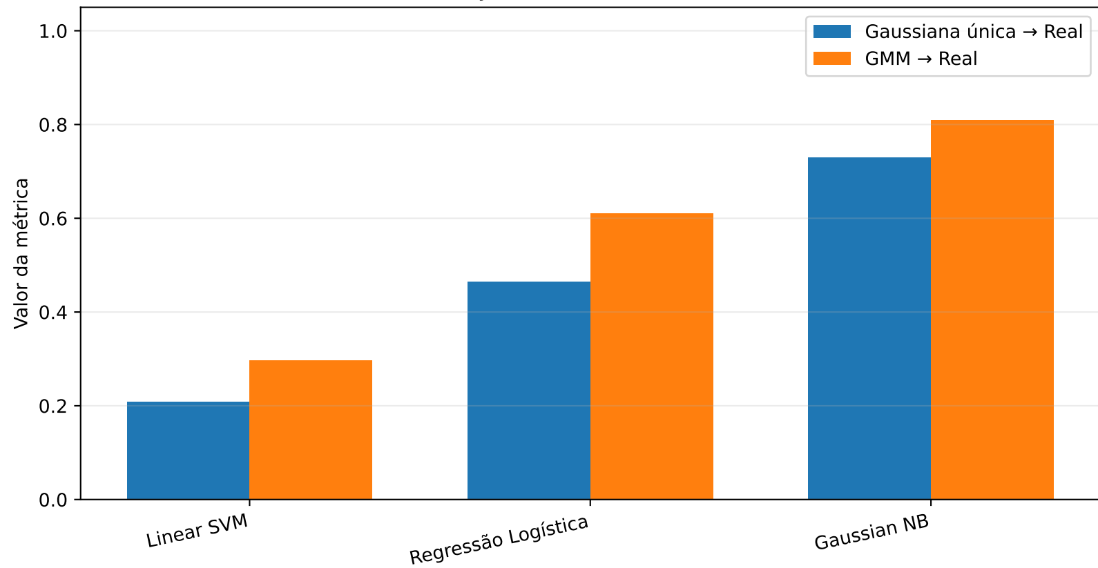
UCI Air Quality: Similaridade de N^* em n = 512
