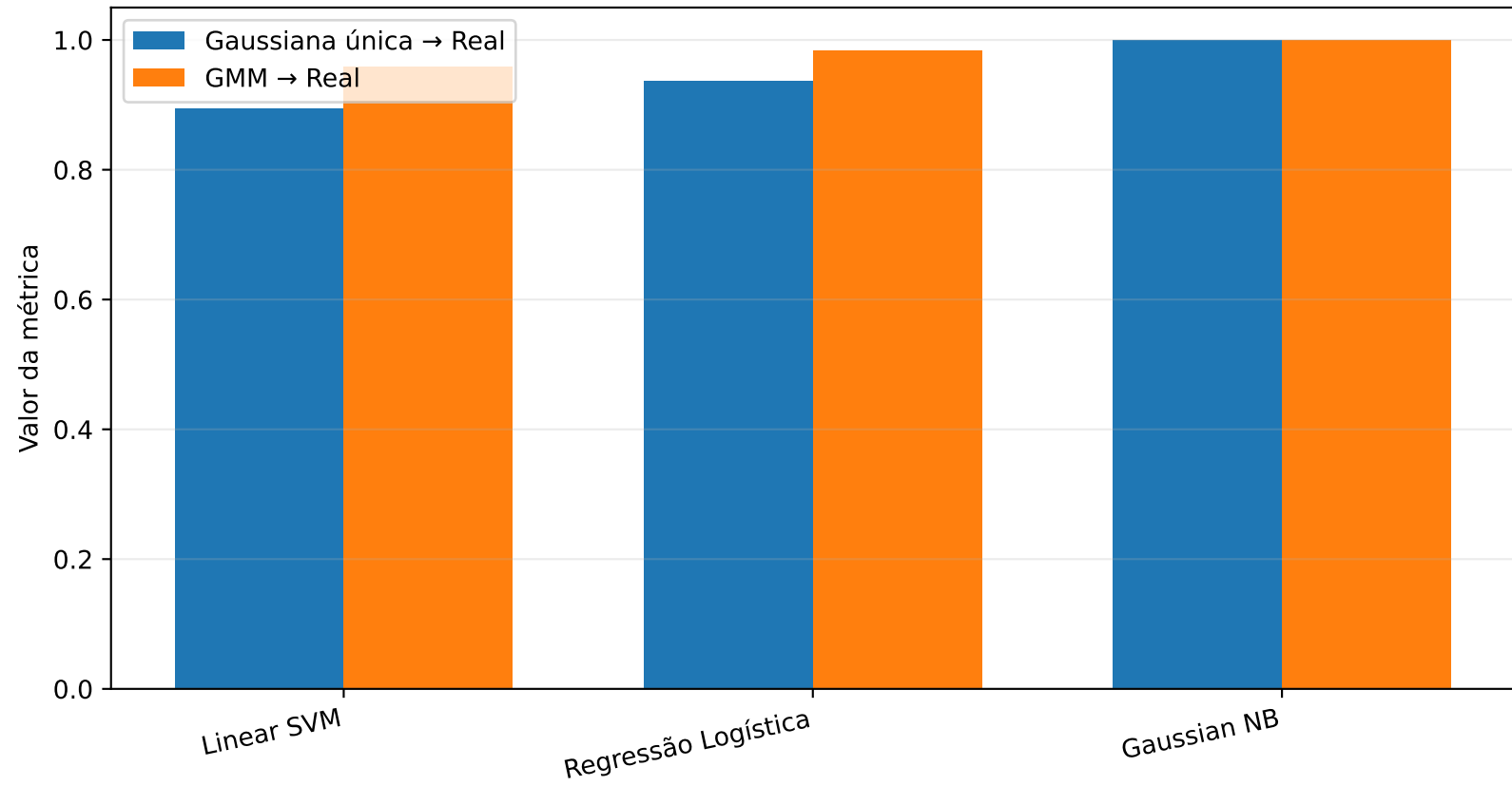
UCI Air Quality: Correlação de ranking em n = 512
