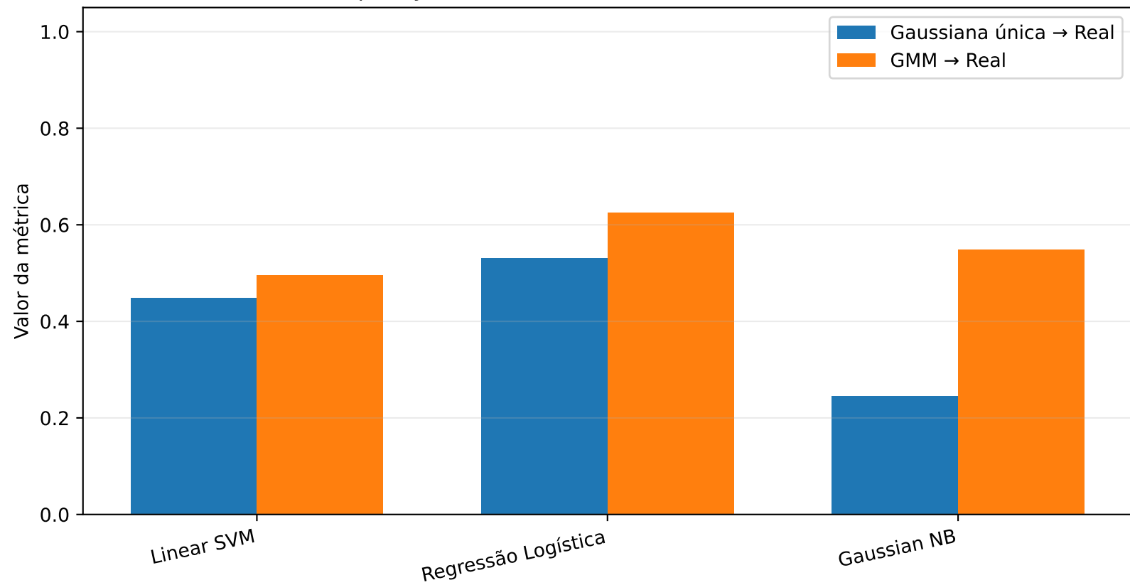
Occupancy Detection: Similaridade de N^* em n = 512
