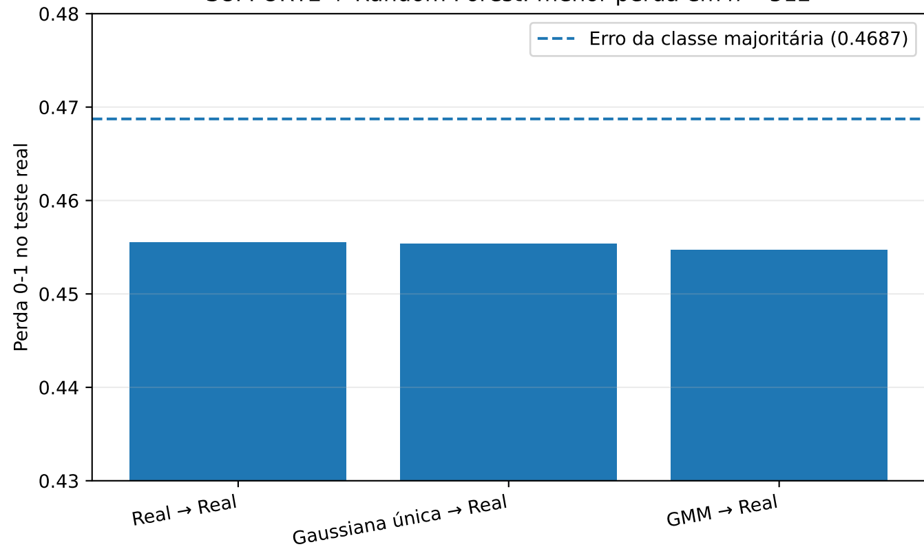
SUPPORT2 + Random Forest: menor perda em n = 512
