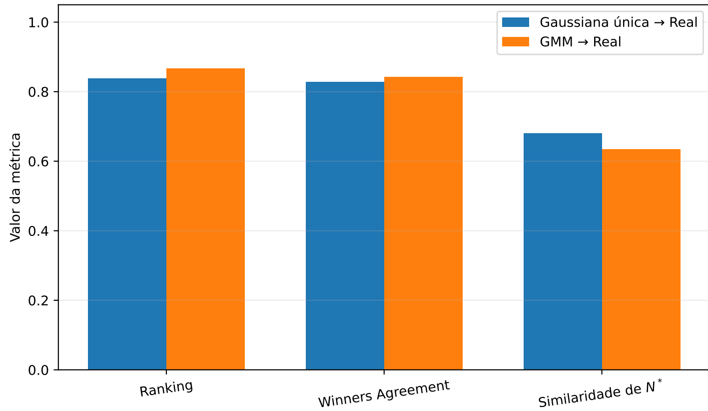
SUPPORT2 + Random Forest: fidelidade estrutural em n = 512
