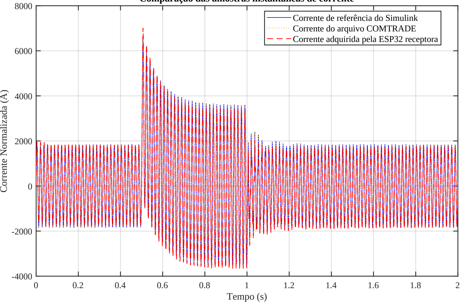
Comparação das amostras instantâneas de corrente
