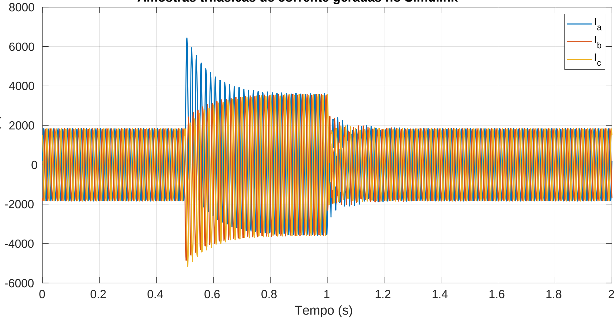
Amostras trifásicas de corrente geradas no Simulink
