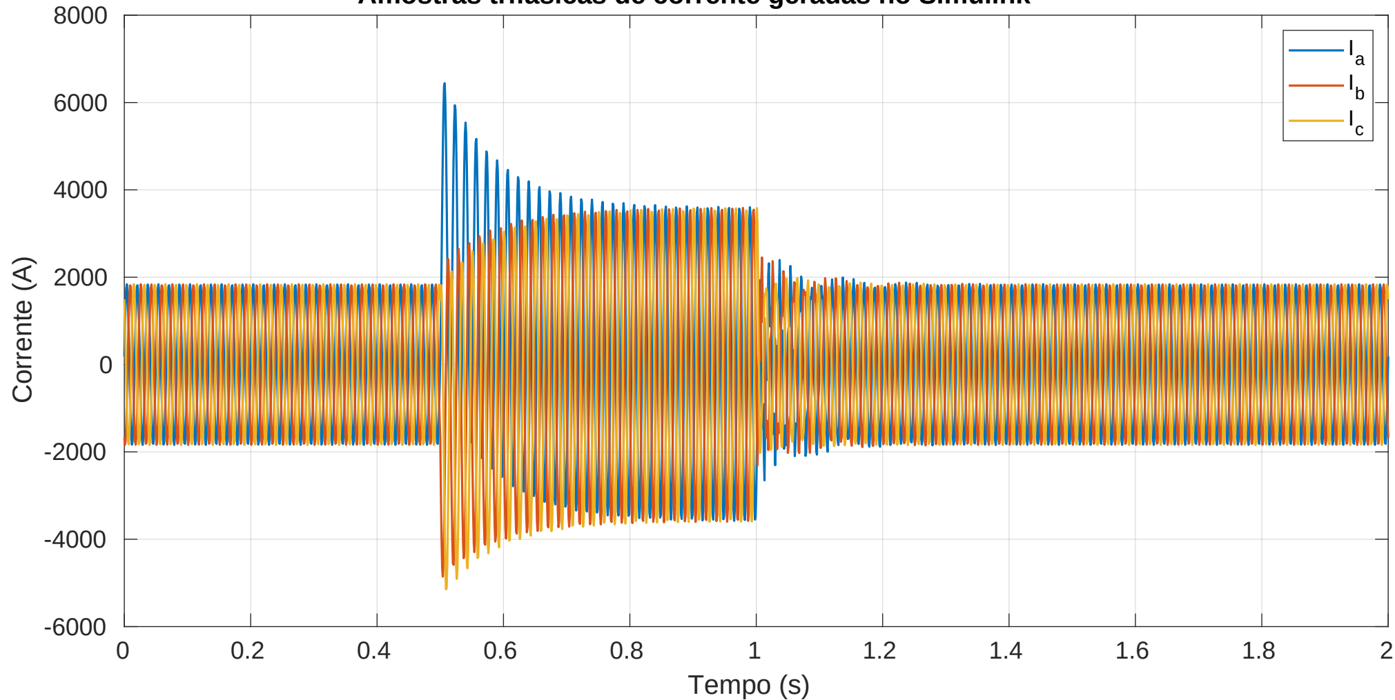
Amostras trifásicas de corrente geradas no Simulink
