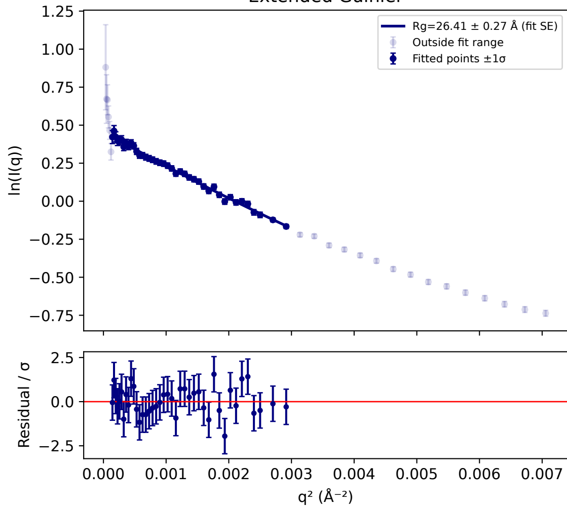
Extended Guinier
