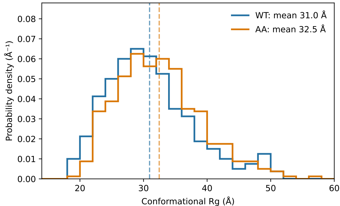
118 residues
