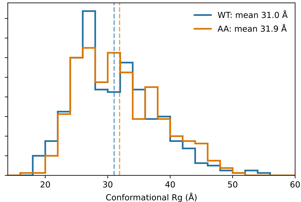
120 residues
