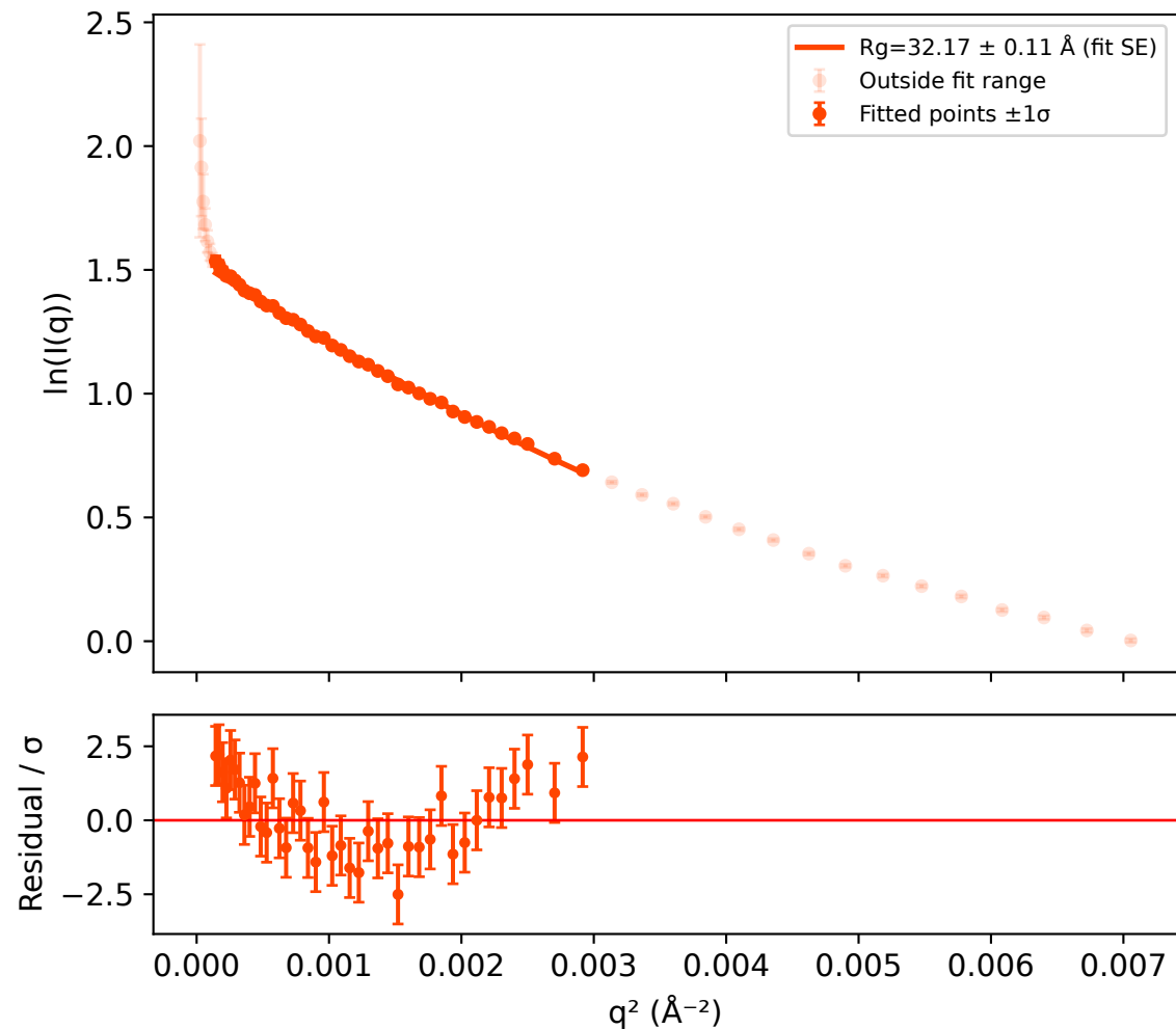
Extended Guinier
