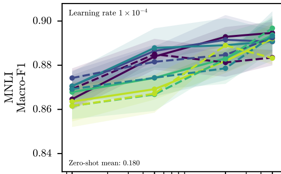
Iso-epoch
