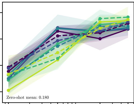
Iso-step
