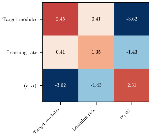
CoNLL-2003
