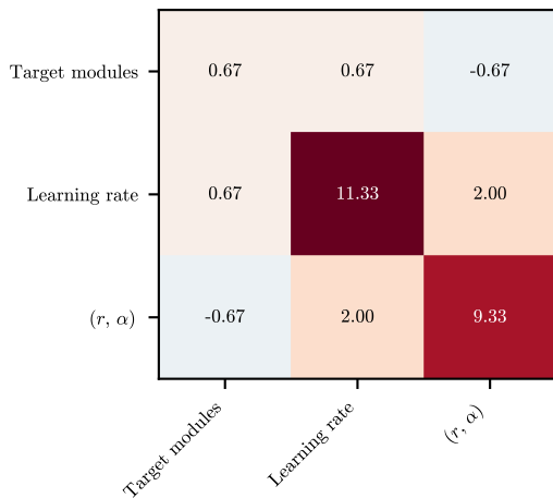
GSM8K
