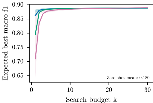
CoNLL-2003
