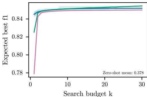
GSM8K
