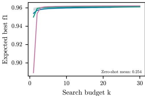
CoNLL-2003
