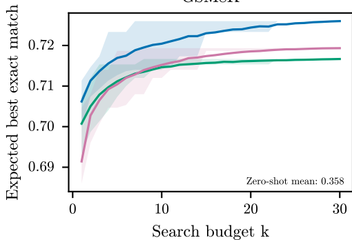
GSM8K
