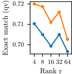
GSM8K
