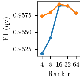
CoNLL-2003
