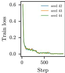
FFT
