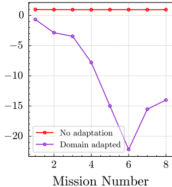
R^2
