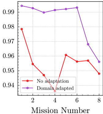
R^2
