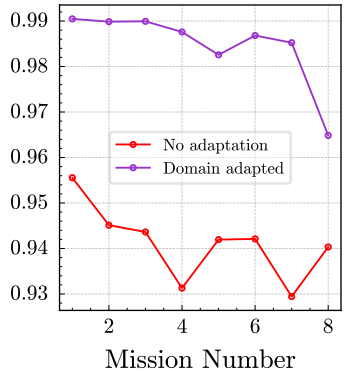
R^2
