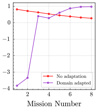
R^2
