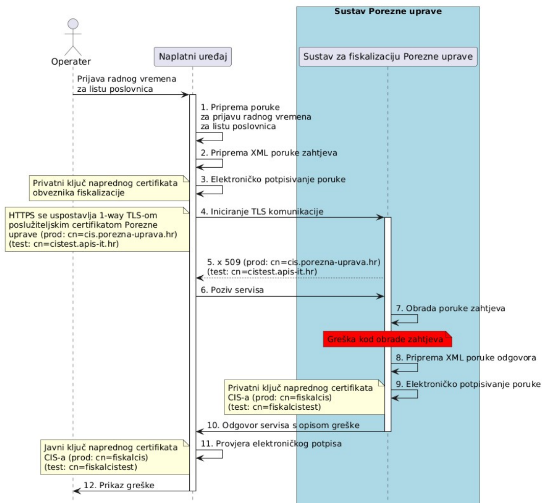
Slika 27. Slijedni dijagram procesa za prijavu radnog vremena za listu poslovnih prostora u slučaju greške na razini ulazne poruke
