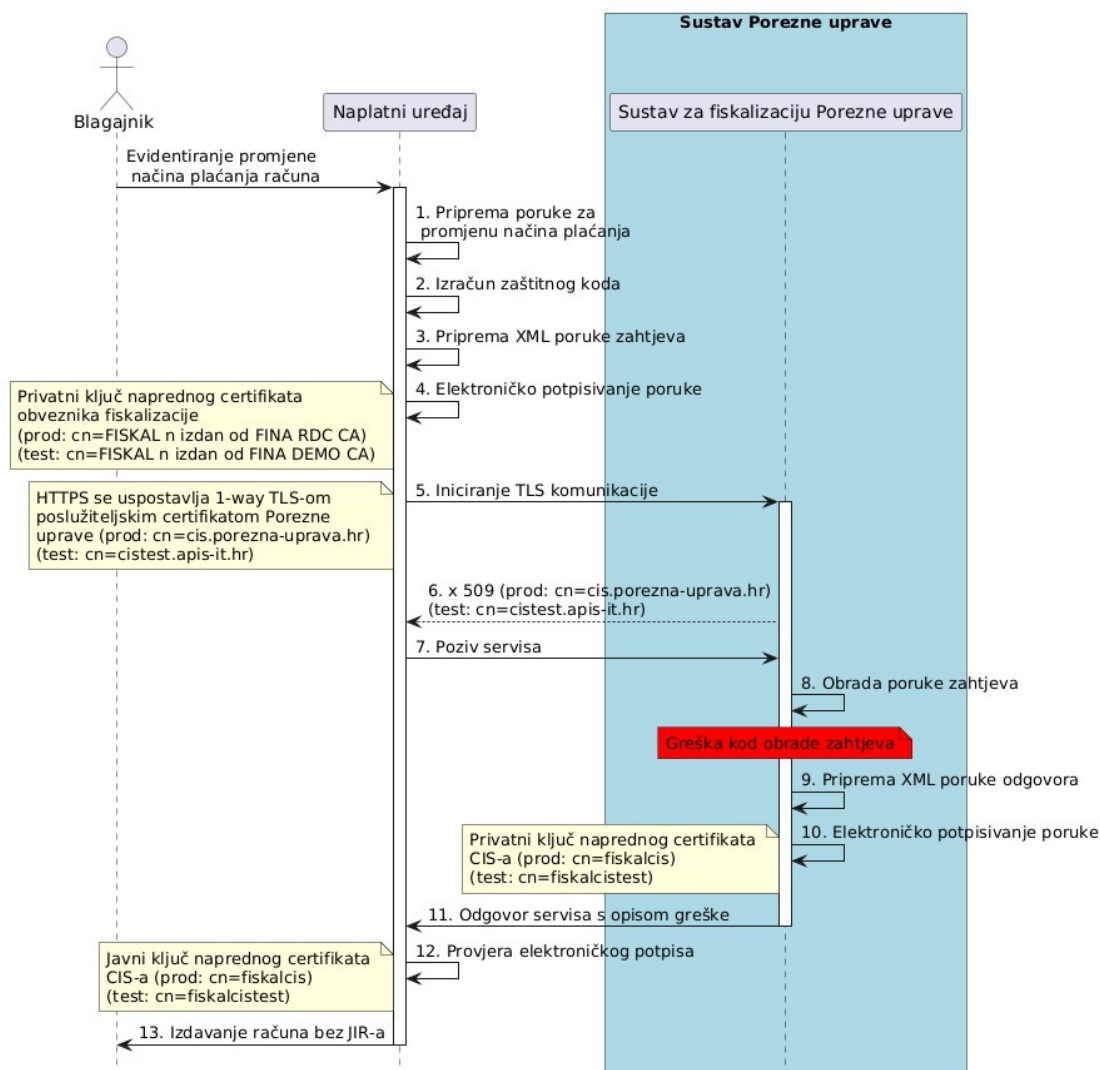
Slika 7. Slijedni dijagram procesa za promjenu načina plaćanja računa u slučaju greške
