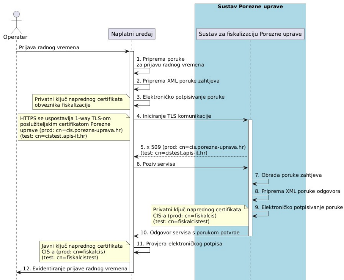
Slika 20. Slijedni dijagram procesa za prijavu radnog vremena
