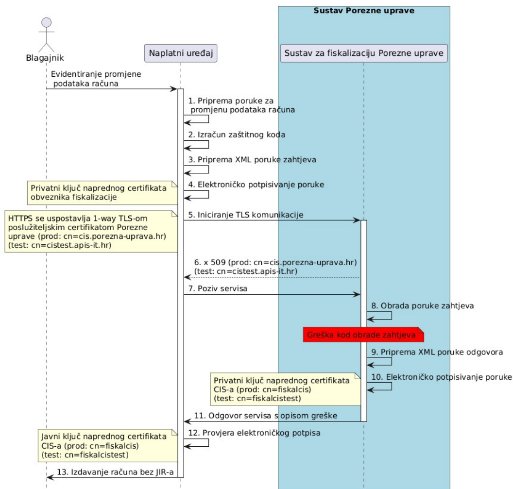
Slika 8. Slijedni dijagram procesa za promjenu podataka računa u slučaju greške
