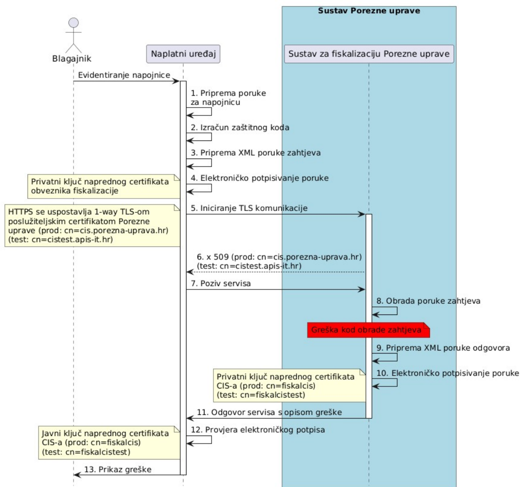
Slika 16. Slijedni dijagram procesa za evidentiranje nagrade za dobro obavljenju uslugu (napojnice) u slučaju greške
