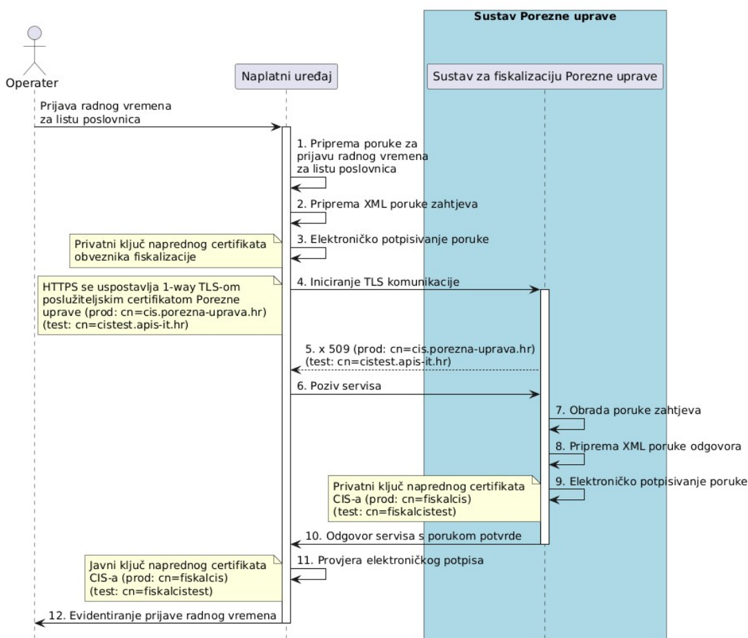
Slika 26. Slijedni dijagram procesa za prijavu radnog vremena za listu poslovnih prostora
