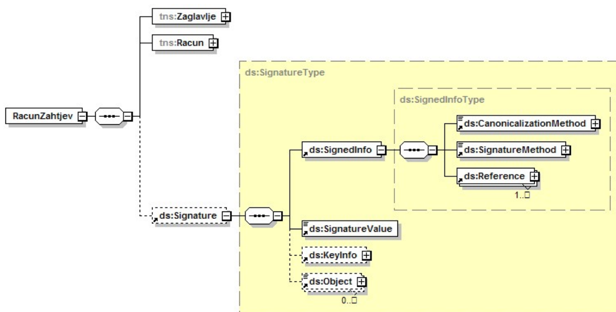
Slika 29. Shema <Signature> elementa
