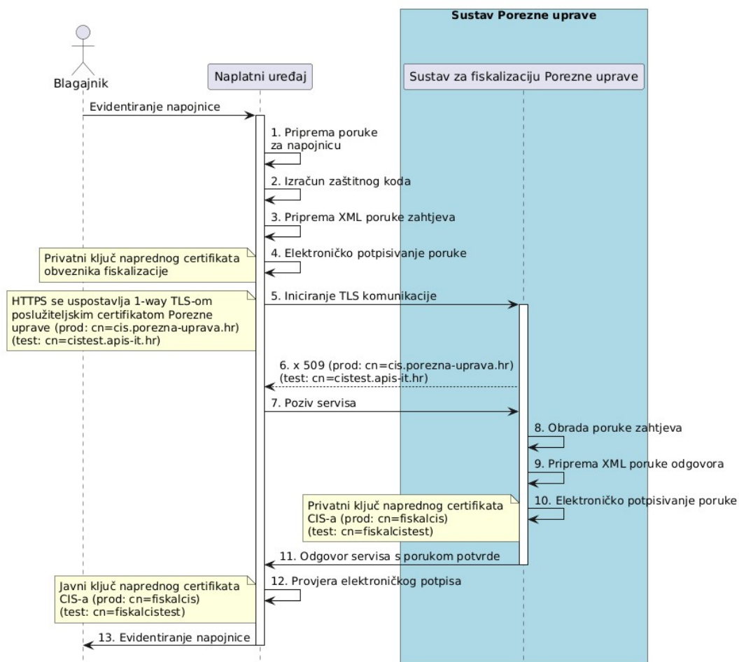
Slika 15. Slijedni dijagram procesa za evidentiranje nagrade za dobro obavljenju uslugu (napojnice)
