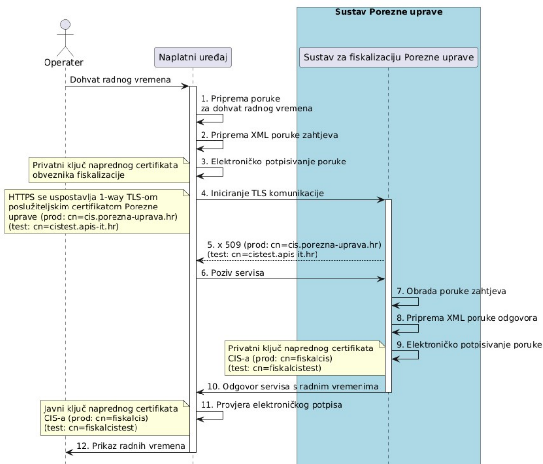
Slika 24. Slijedni dijagram procesa za dohvat radnog vremena
