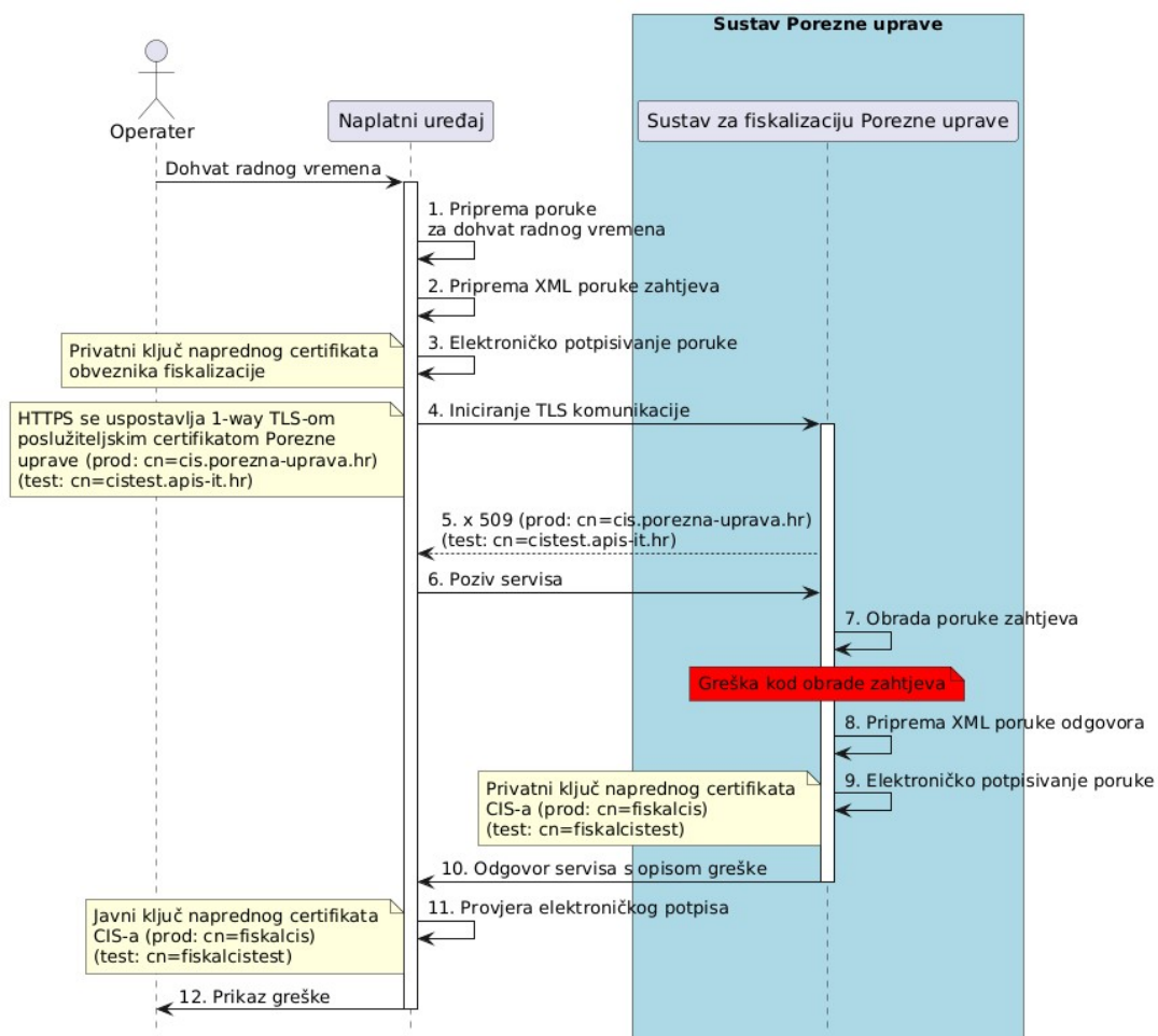
Slika 25. Slijedni dijagram procesa za dohvat radnog vremena u slučaju greške
