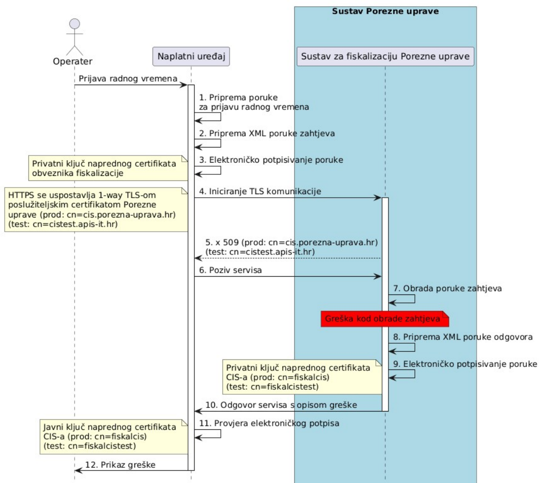
Slika 21. Slijedni dijagram procesa za prijavu radnog vremena u slučaju greške
