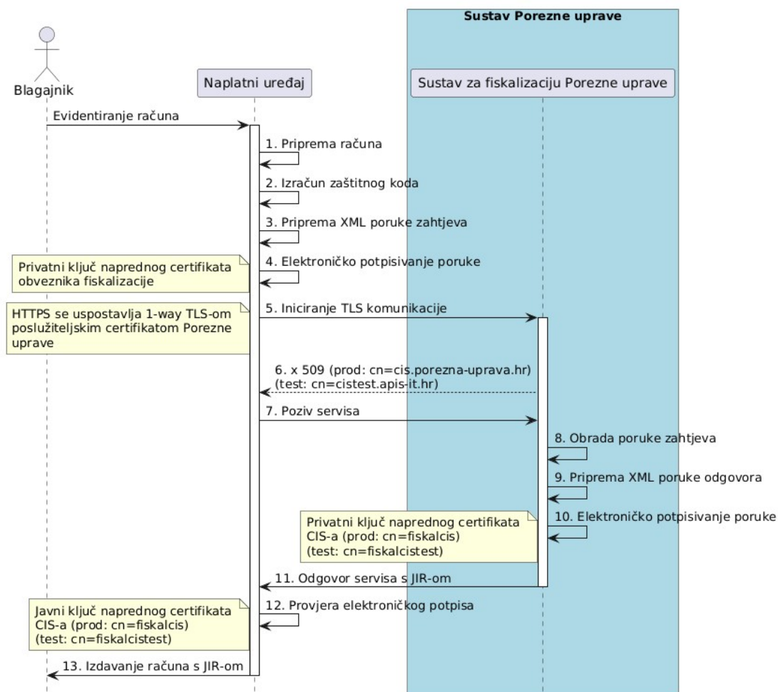
Slika 1. Slijedni dijagram procesa za slanje računa
