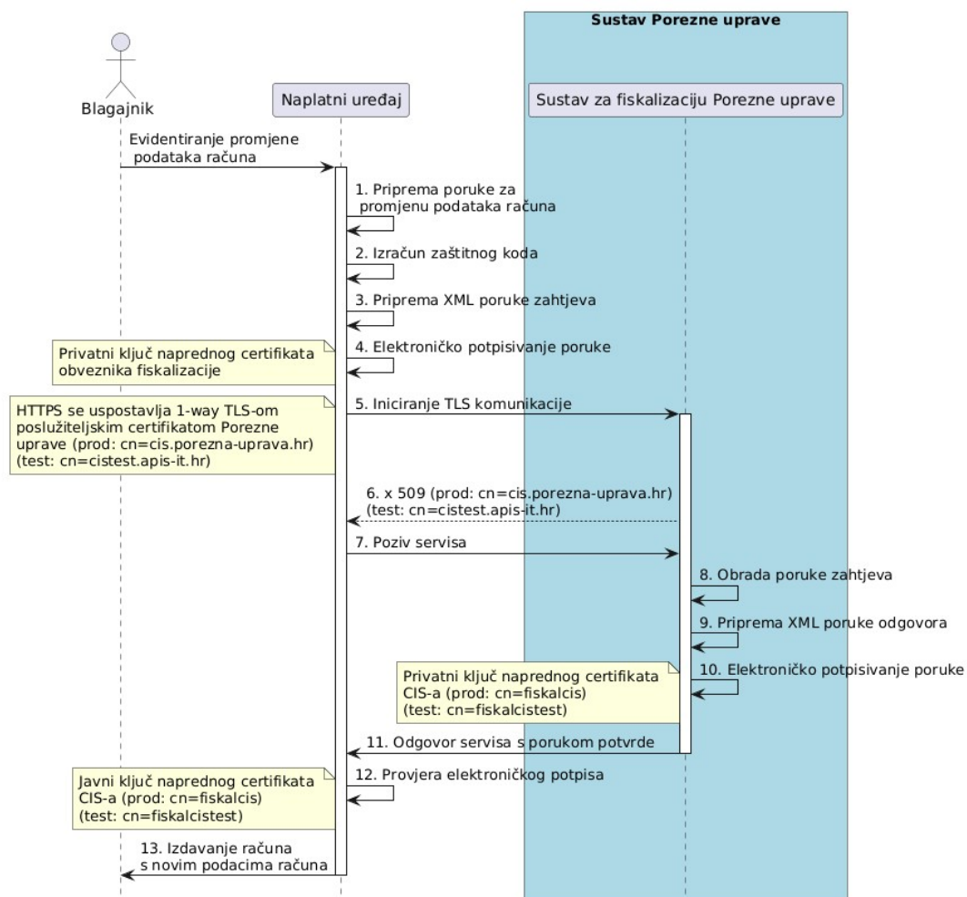
Slika 6. Slijedni dijagram procesa za promjenu podataka računa
