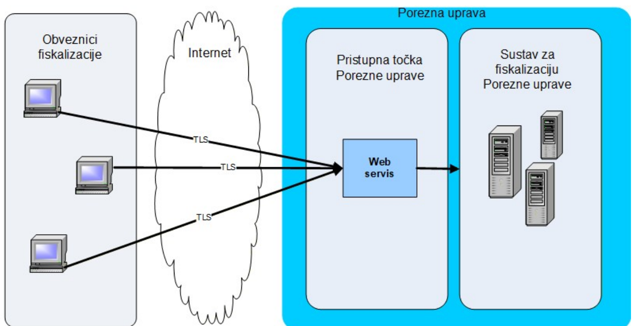
Slika 28. Topologija pristupa Sustavu za fiskalizaciju Porezne uprave
