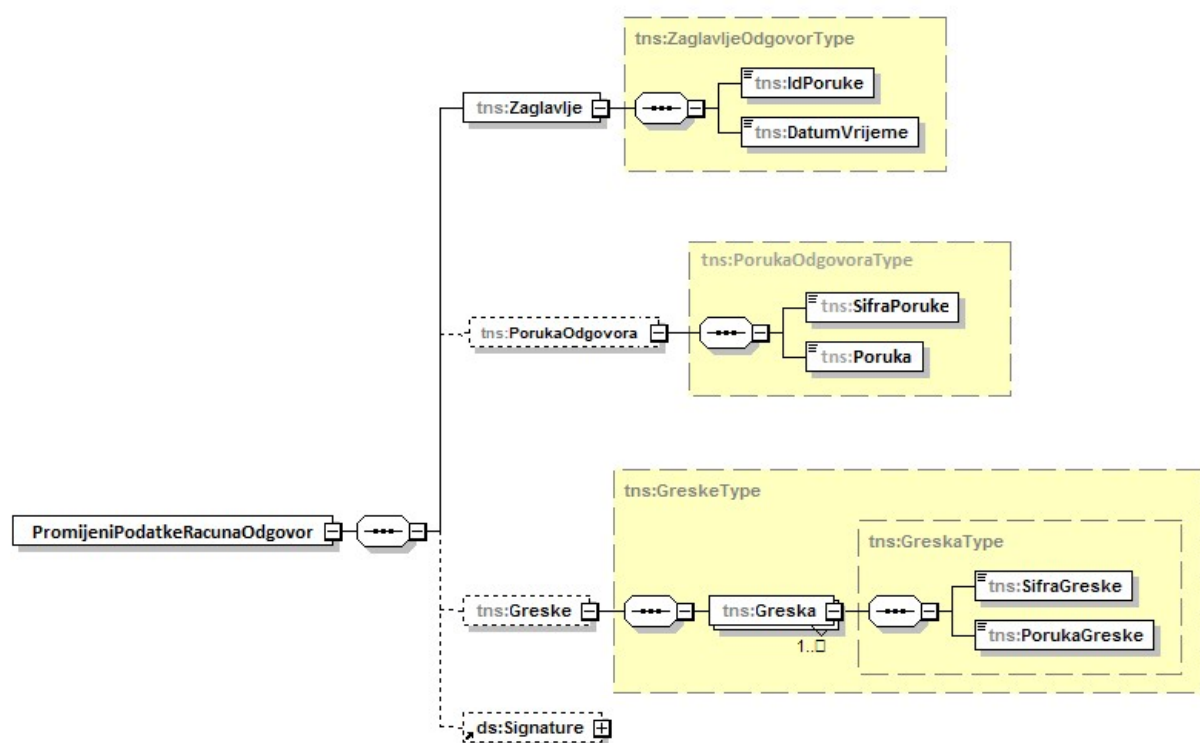
Slika 12. Shema poruke odgovora za promjenu podataka računa
