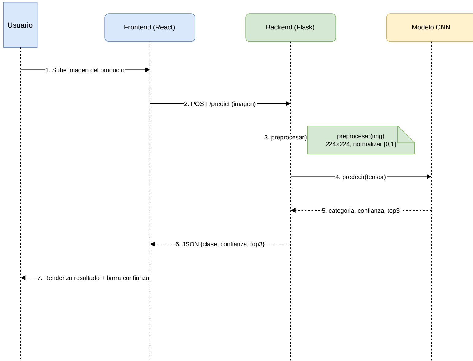
Figura 3. Diagrama de Secuencia: flujo de clasificación.
