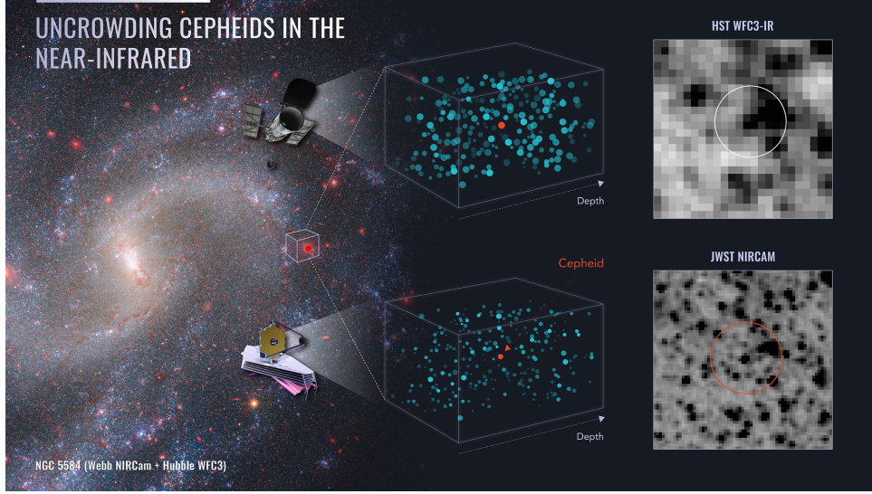
Figura 1.1: Imagen mostrando la galaxia NGC 5584. La visualización ilustra cómo el telescopio Webb (NIRCam) logra separar una estrella Cefeida (punto naranja) de la multitud de estrellas de fondo (puntos azules), una distinción que la menor resolución del Hubble (WFC3-IR) en el infrarrojo cercano no permitía hacer con claridad, como se ve en los recuadros ampliados. Imagen tomada de NASA et al. (2023)
