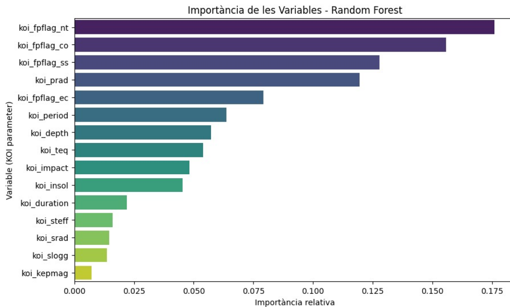
Figura 7: Gràfic d'importància relativa de les variables per al model Random Forest òptim.
