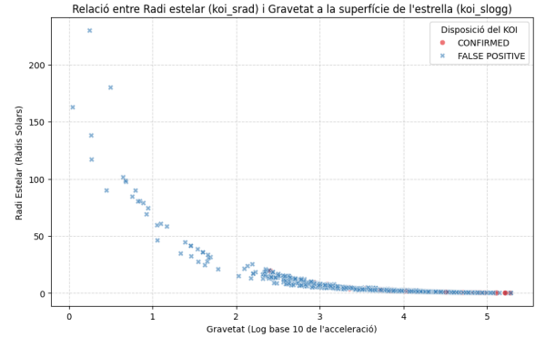
(b) Relació entre radi estel·lar i gravetat a la superfície de l'estrella
