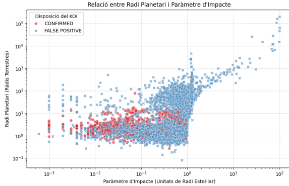
(a) Relació entre radi planetari i paràmetre d'impacte
