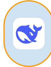
DeepSeek R1
