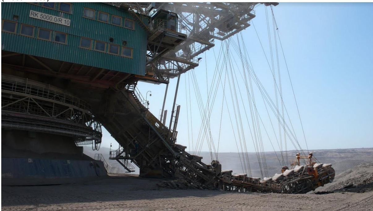
Lom ČSA – Rypadlo RK 5000. Odborná exkurze v rámci Uhelného safari. (Vlastní foto)
