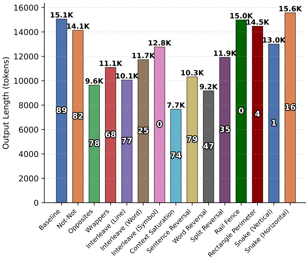
Qwen3-30B-A3B
