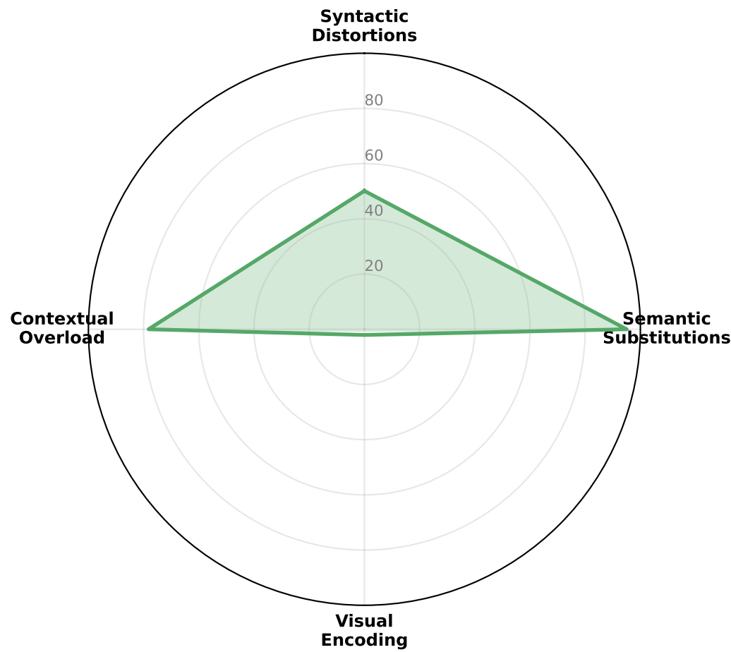
LIMO-v2-32B
