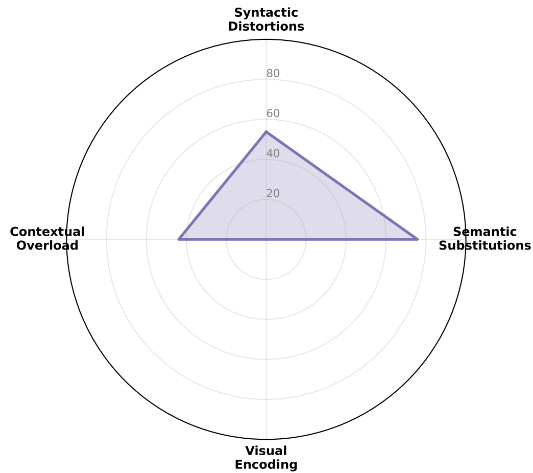
Qwen3-30B-A3B
