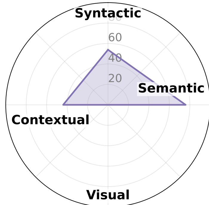
Qwen3-30B-A3B
