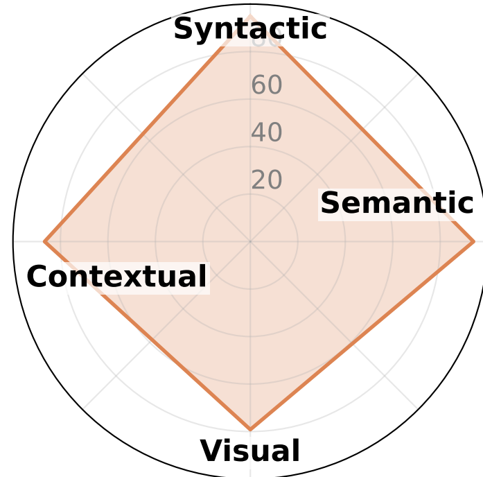
Nemotron-32B
