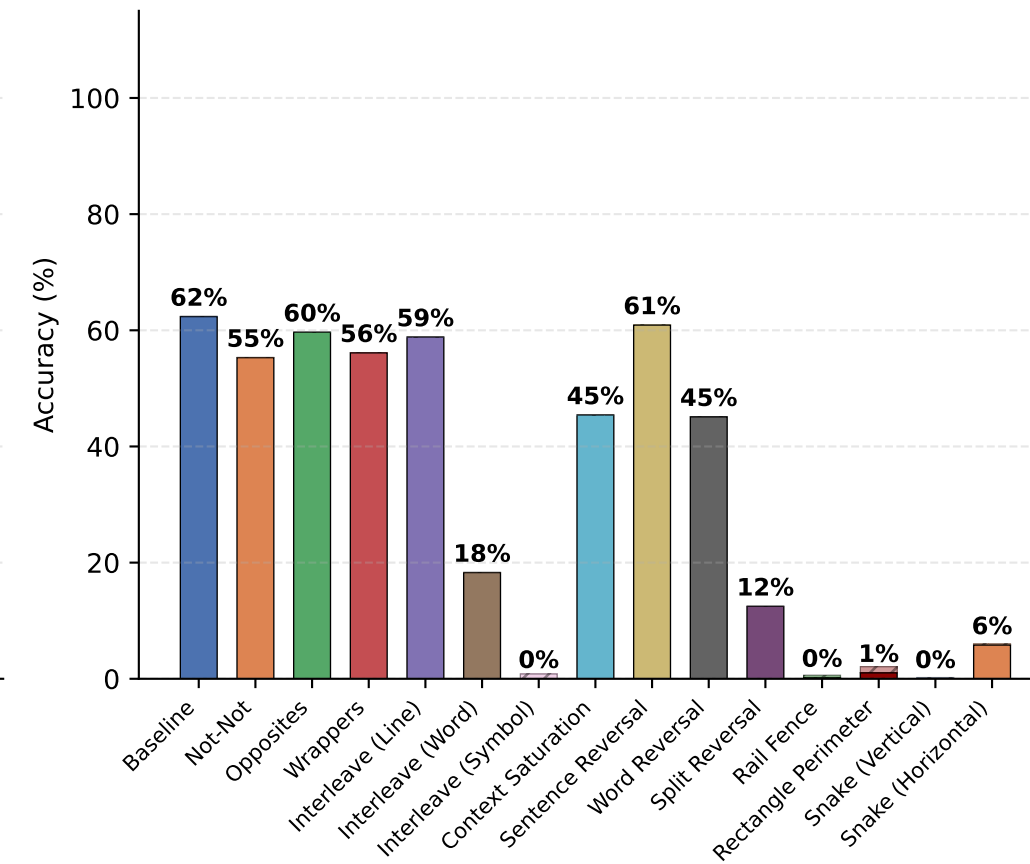
LIMO-v2-32B
