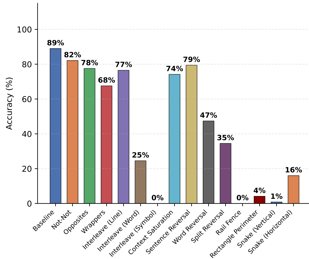
Qwen3-30B-A3B
