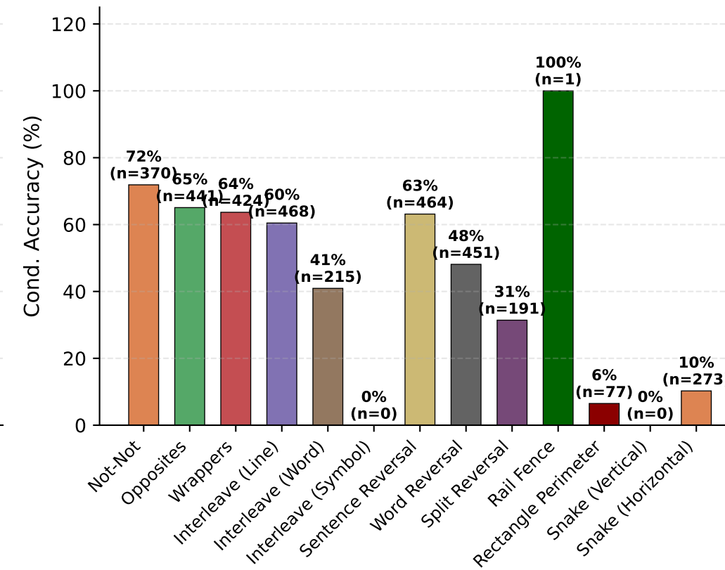
LIMO-v2-32B
