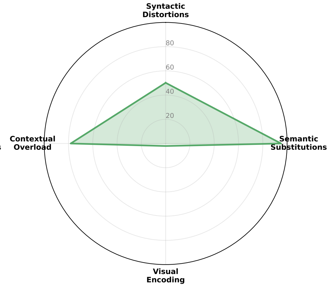
LIMO-v2-32B
