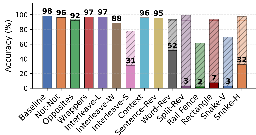
Qwen3-30B-A3B
