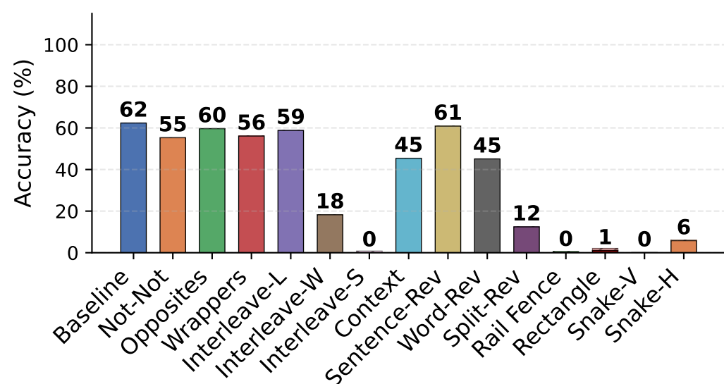
LIMO-v2-32B
