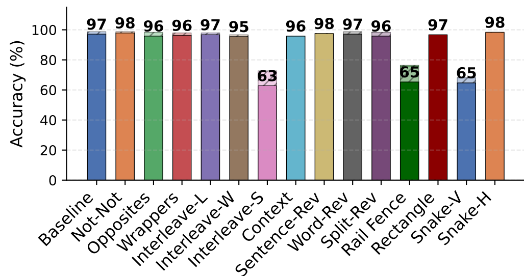
Claude Opus 4-6
