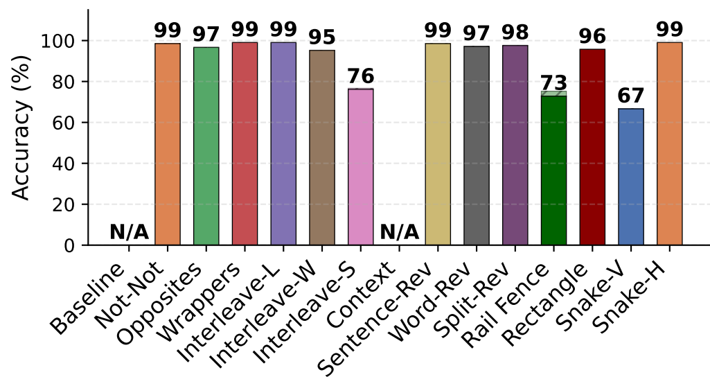
Nemotron-32B
