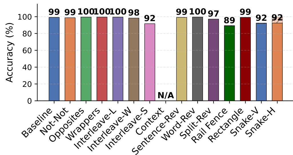
Claude Opus 4.6
