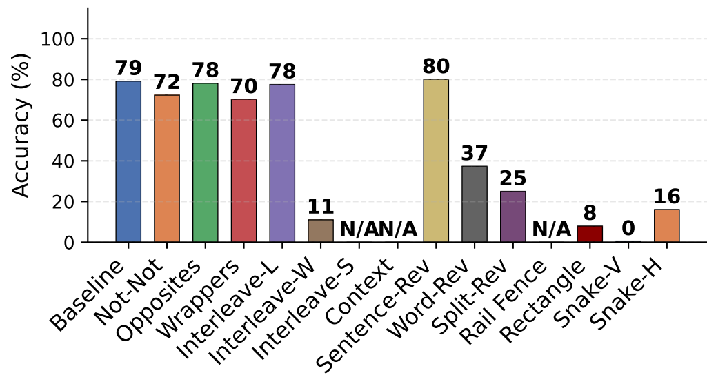
Qwen3-30B-A3B
