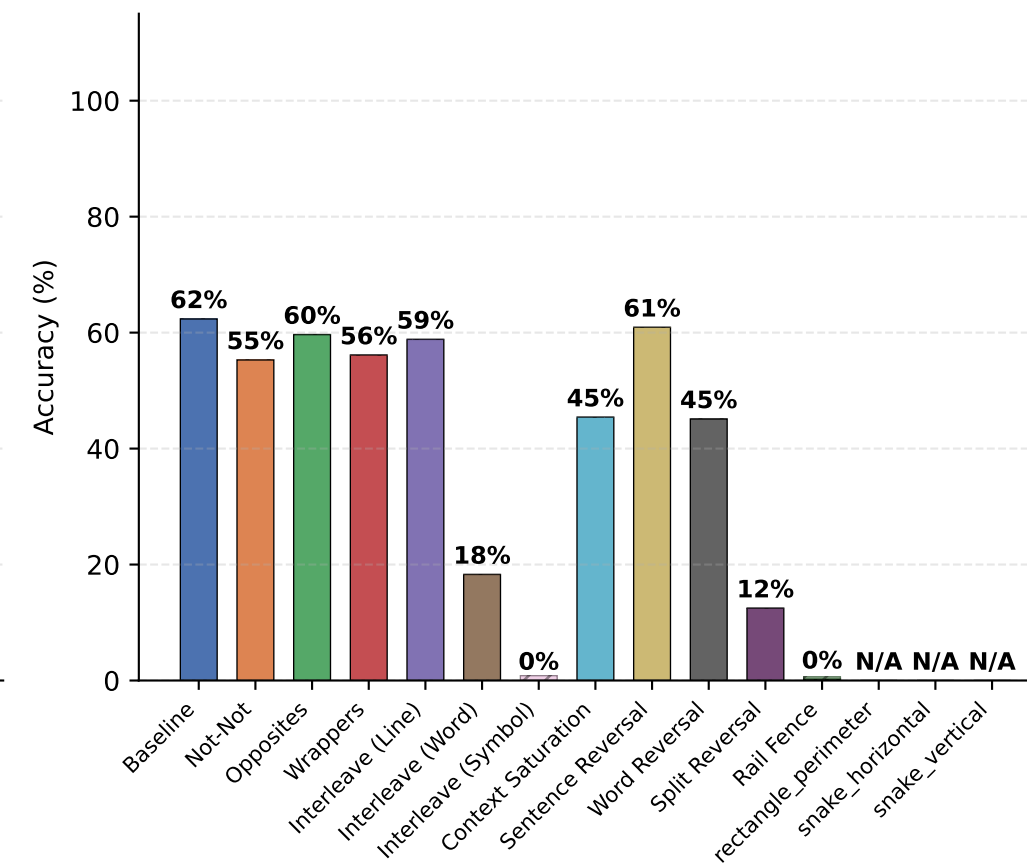
LIMO-v2-32B
