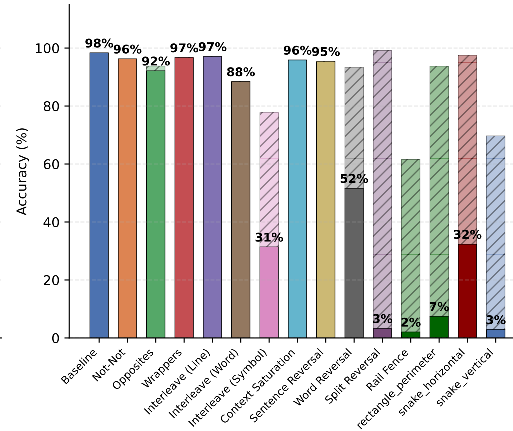
LIMO-v2-32B
