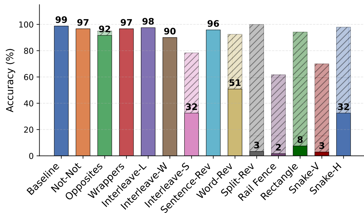
Opus 4.6
