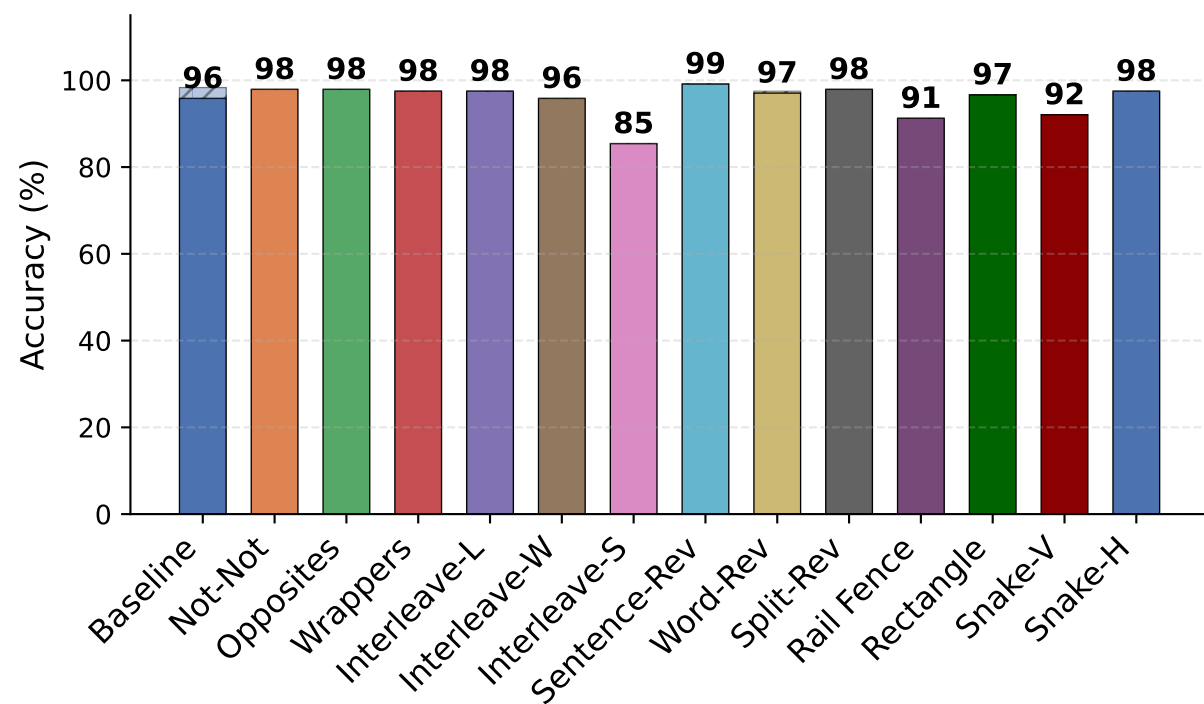
GPT-5.4
