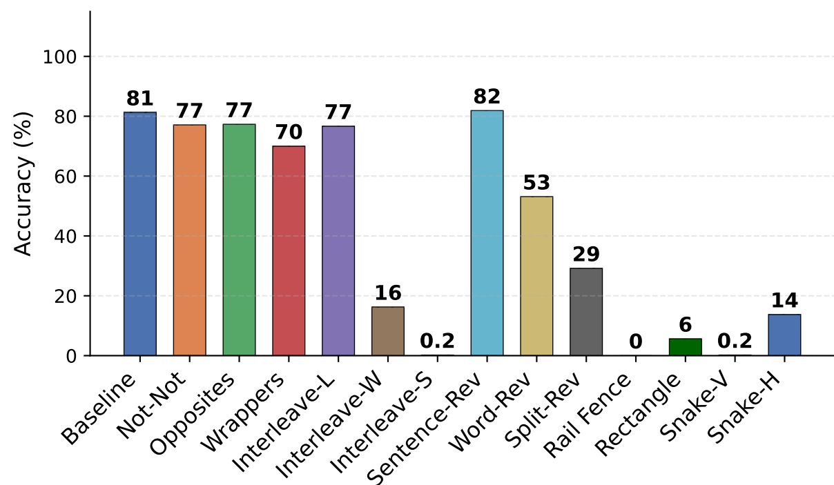
Nemotron-32B
