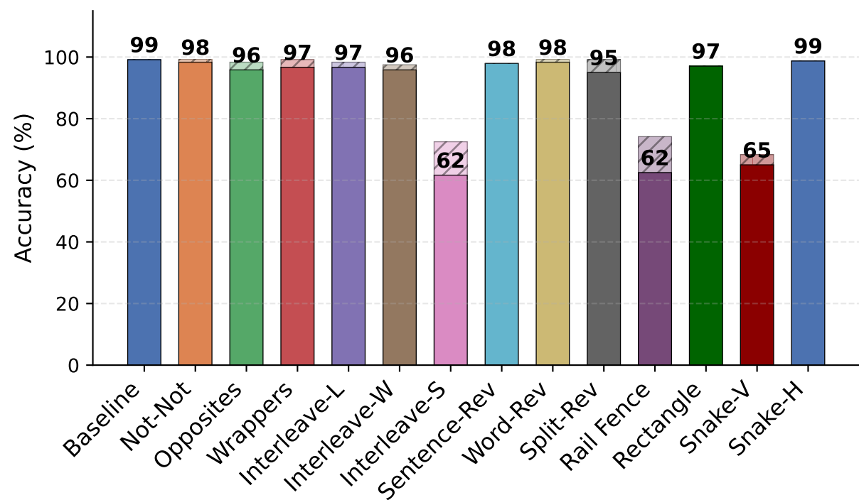
Gemini 3.1 Pro
