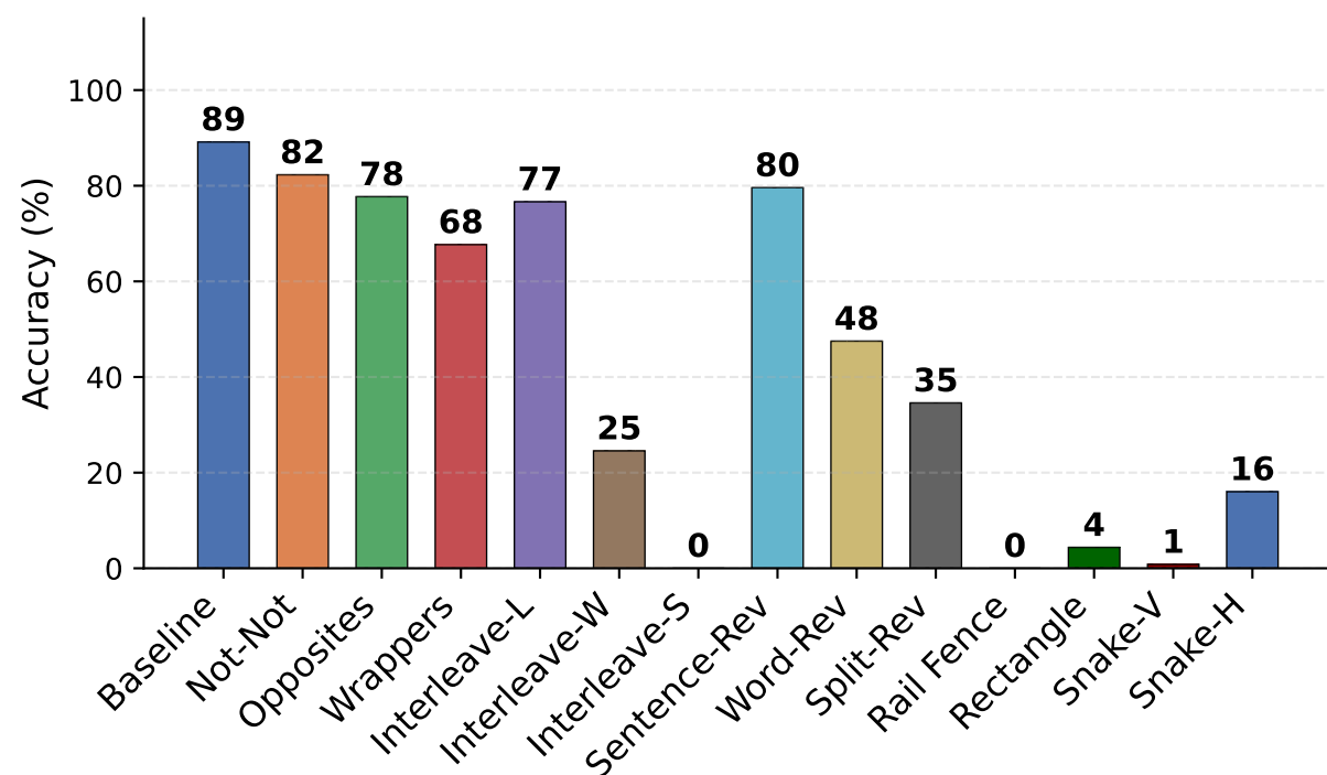
Qwen3-30B-A3B
