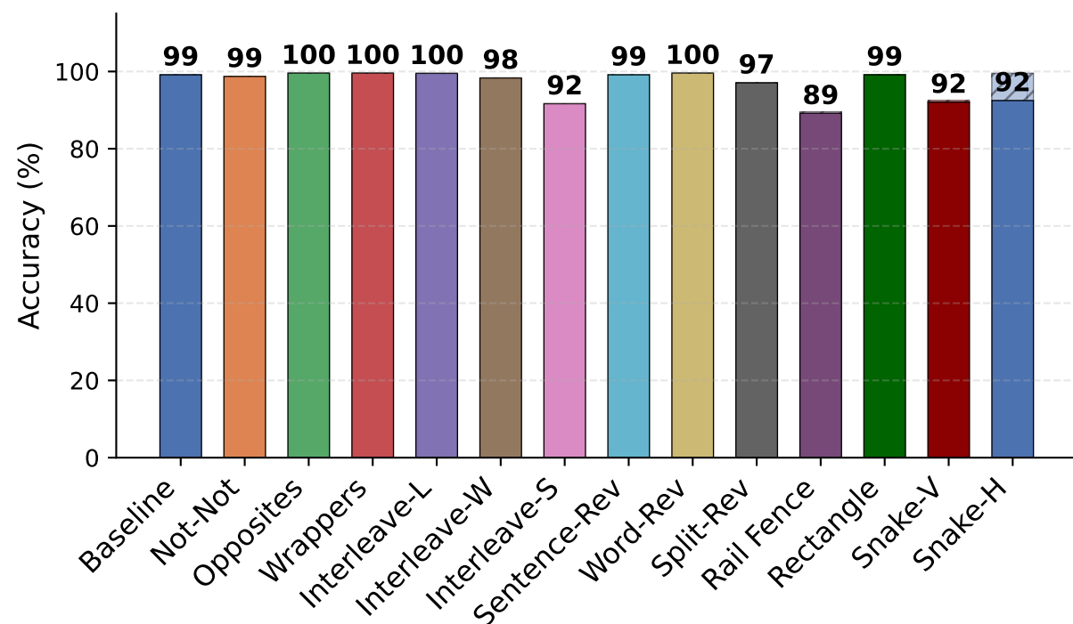
GPT-5.4
