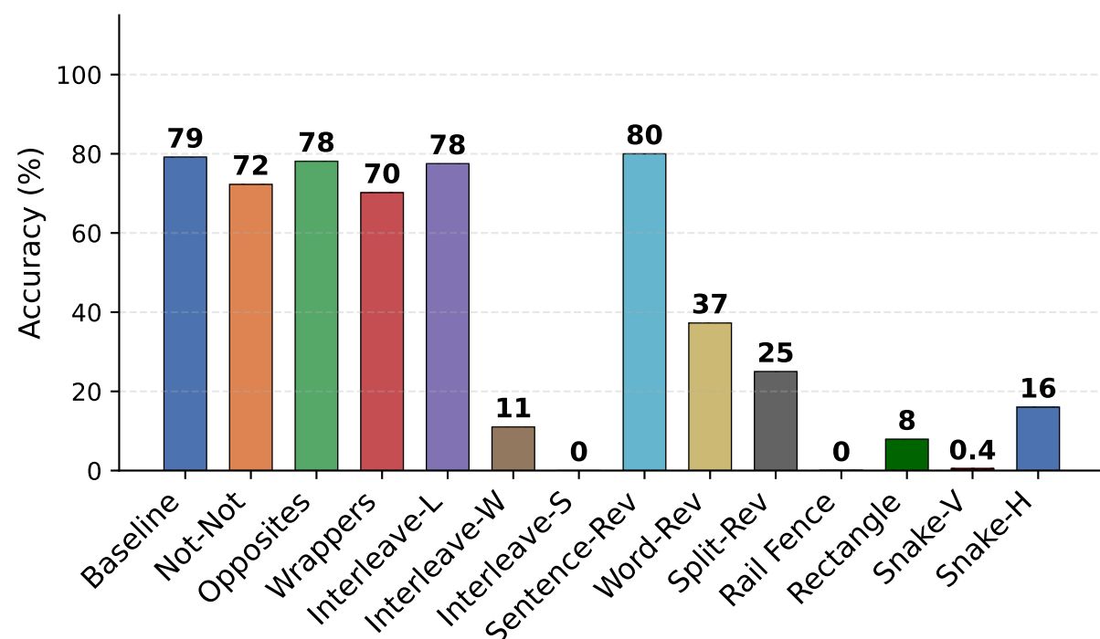
Nemotron-32B
