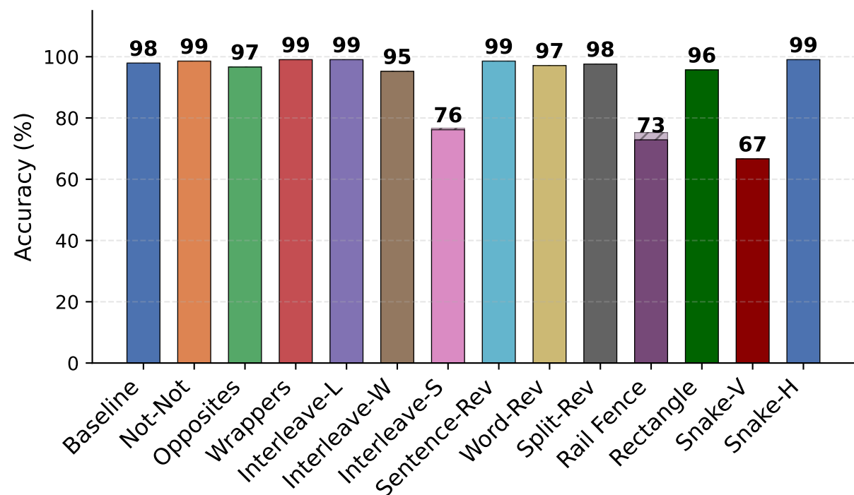
Gemini 3.1 Pro
