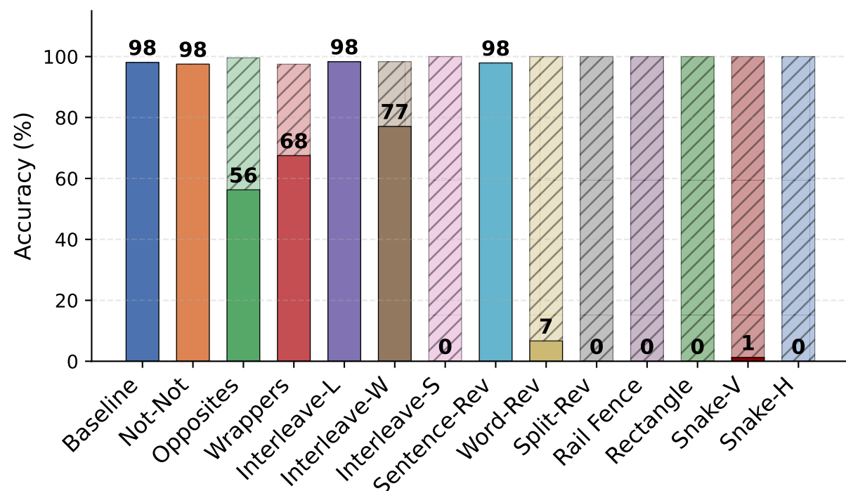
Opus 4.6
