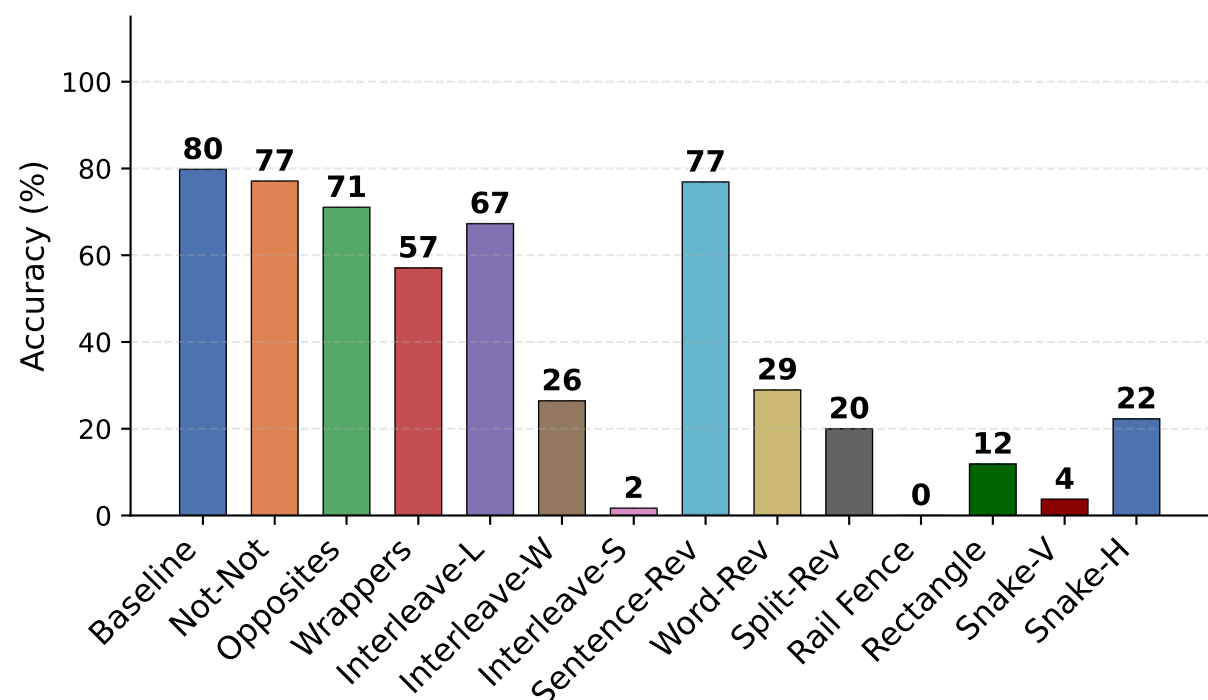
Qwen3-30B-A3B
