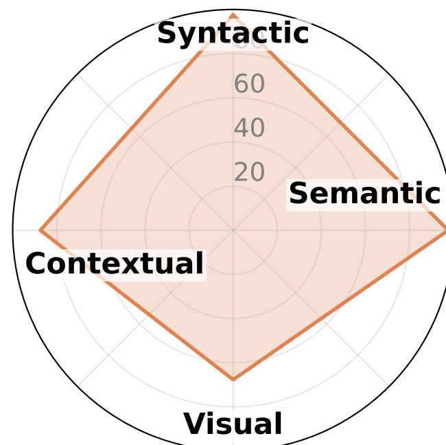
Nemotron-32B
