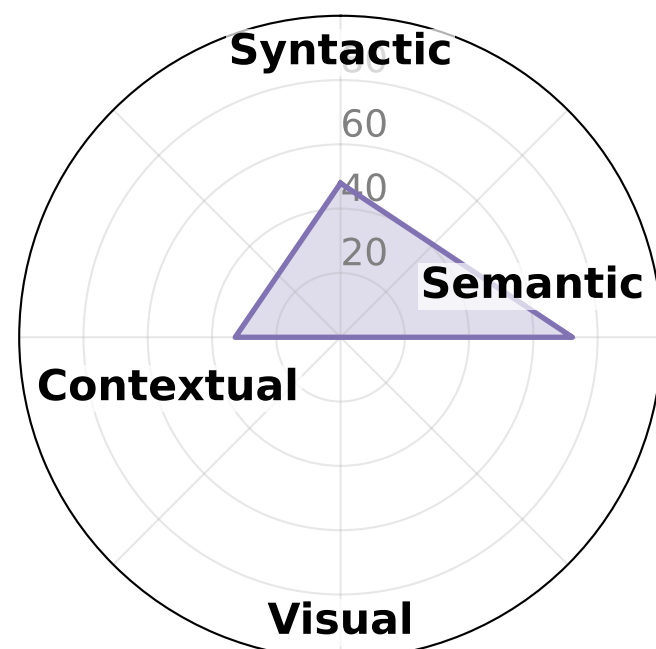
Qwen3-30B-A3B
