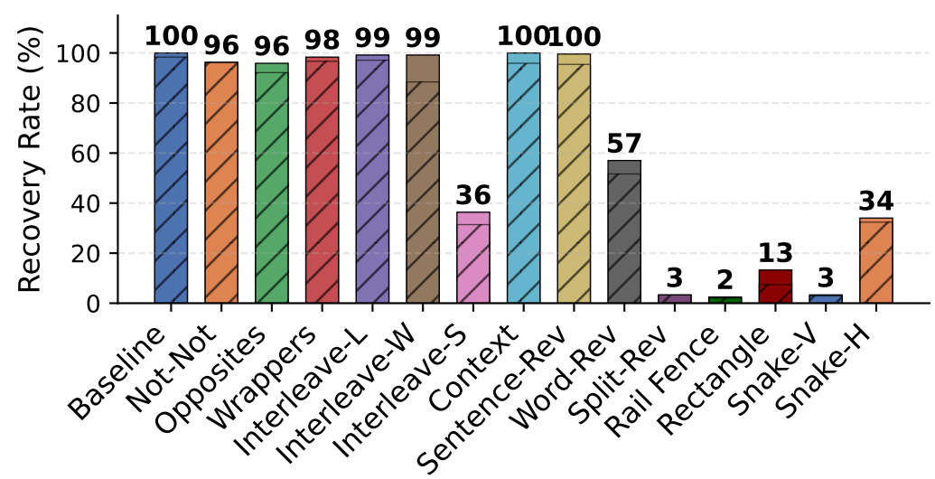
Claude Opus 4-6
