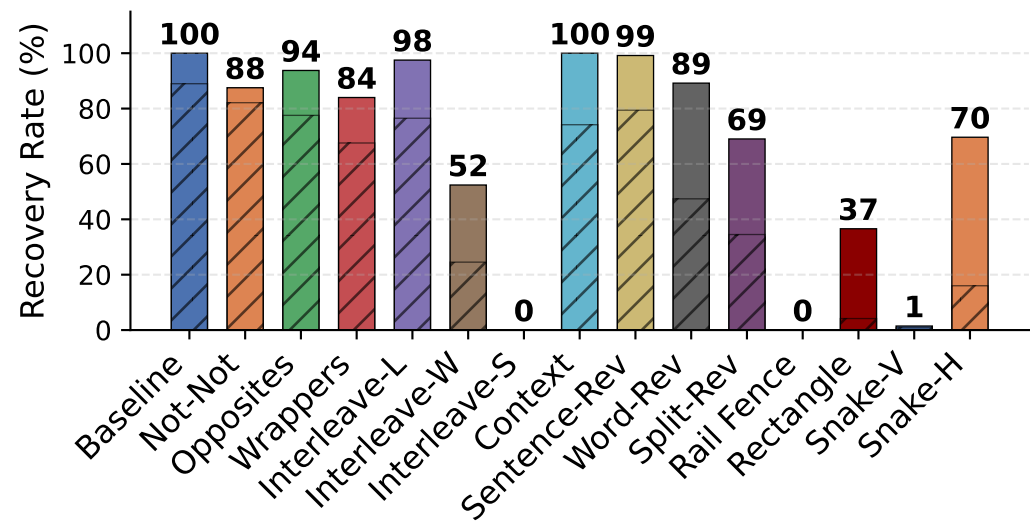
LIMO-v2-32B
