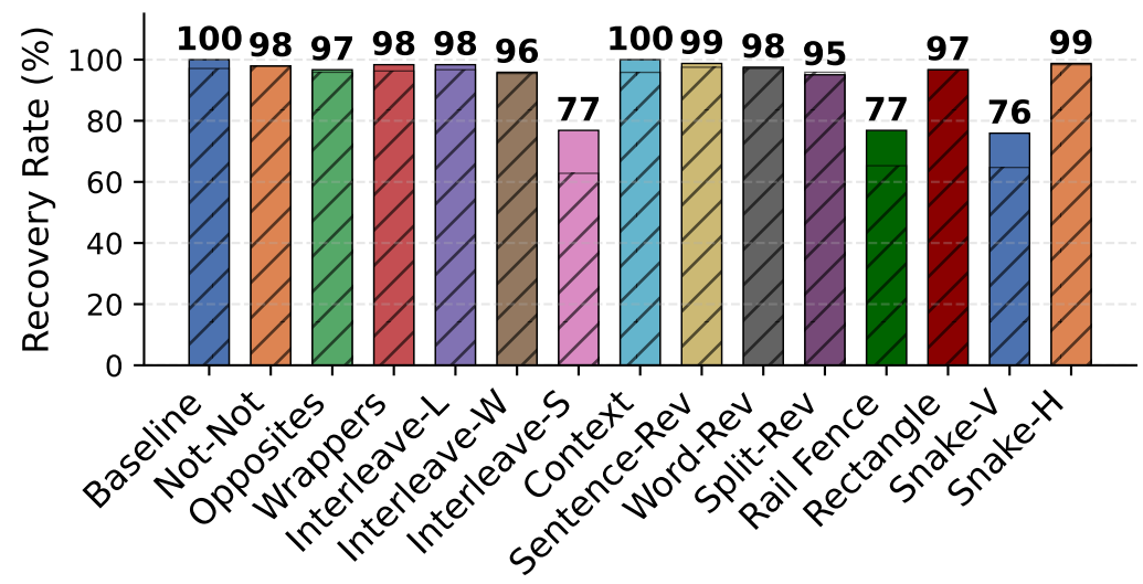
Claude Opus 4-6
