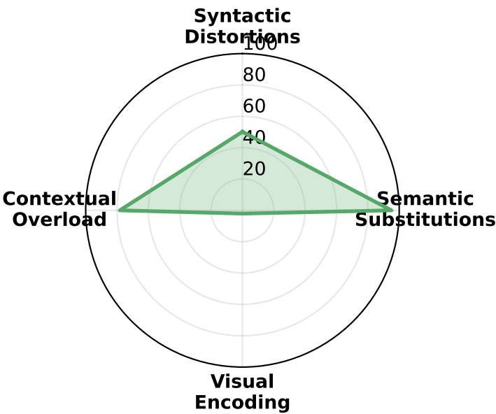
Qwen3-30B-A3B
