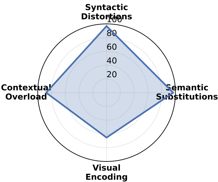
Claude Opus 4-6
