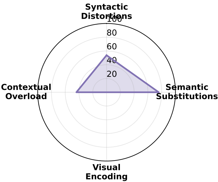
LIMO-v2-32B
