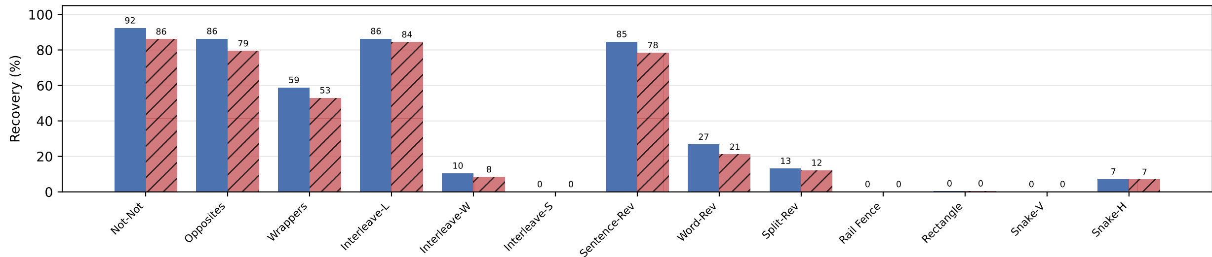
Qwen3-30B-A3B
