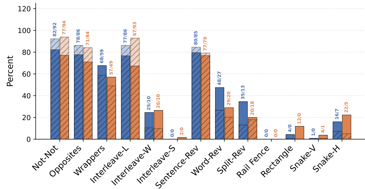
Qwen3-30B-A3B
