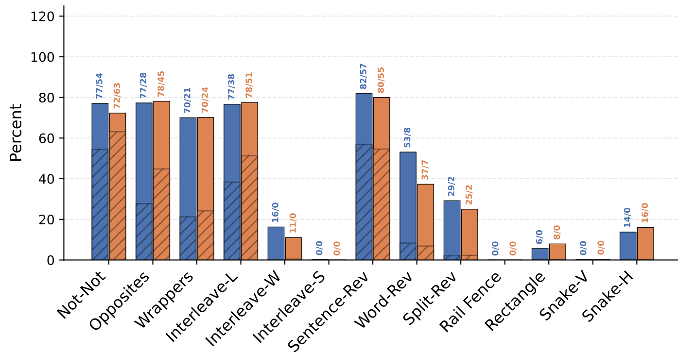
Nemotron-32B
