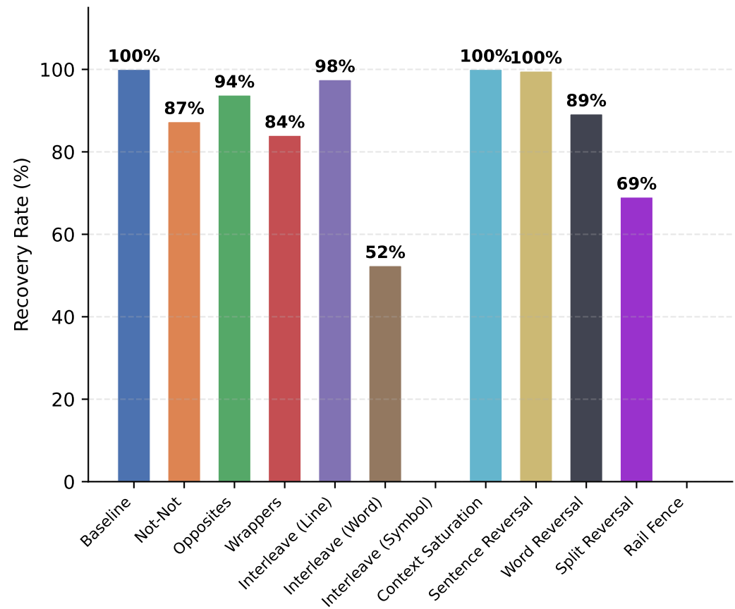
Qwen3-30B
