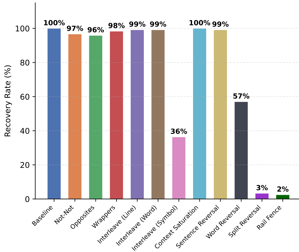
LIMO-v2 (32B)
