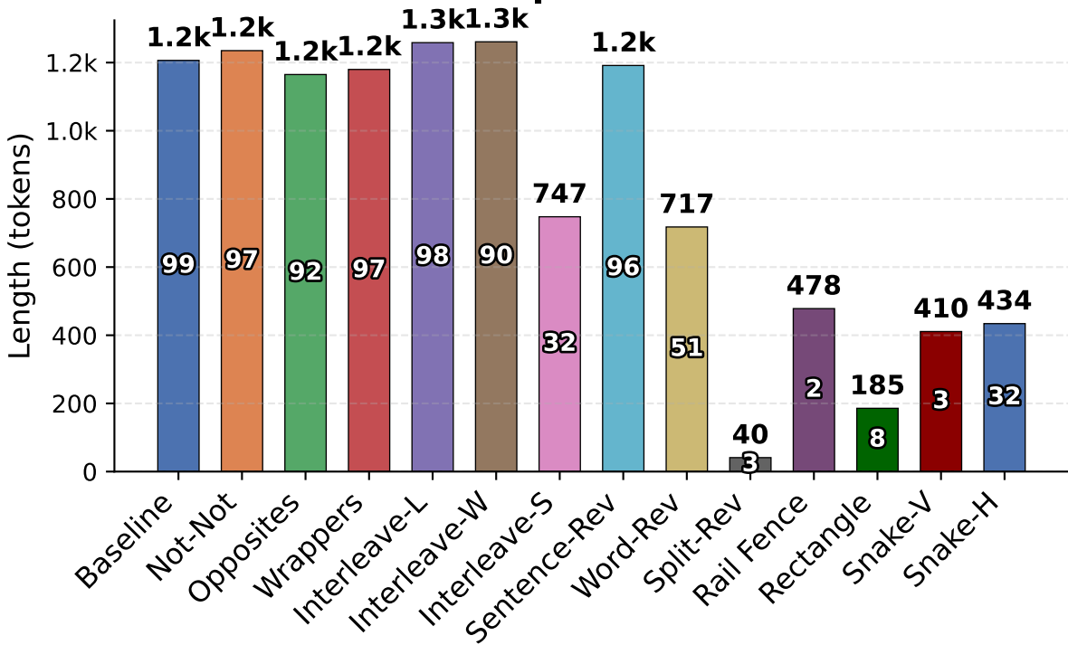
Opus 4.6
