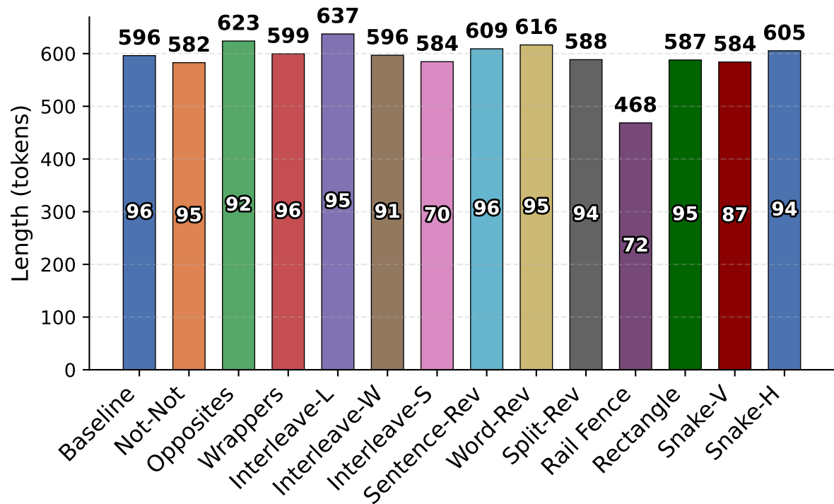
GPT-5.4
