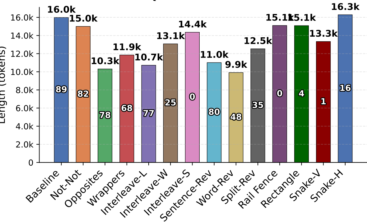
Qwen3-30B-A3B
