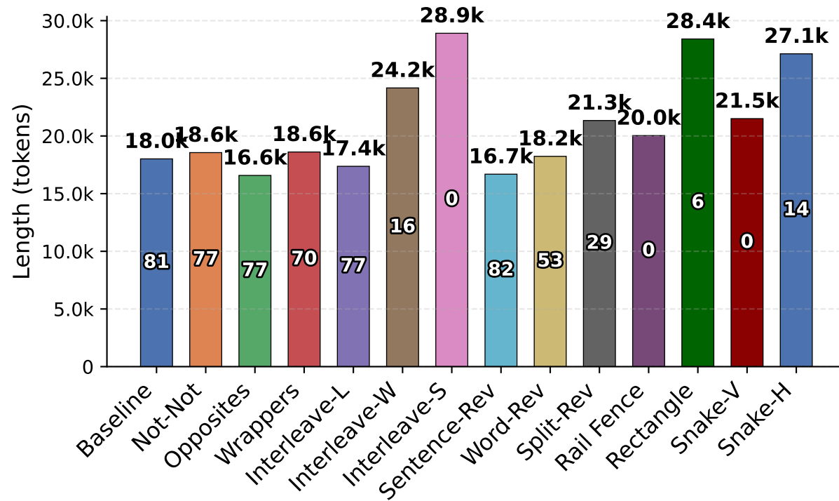
Nemotron-32B
