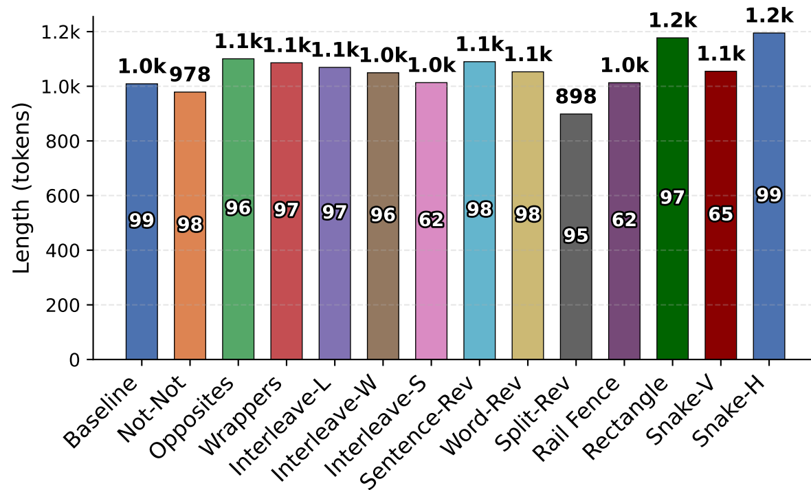
Gemini 3.1 Pro
